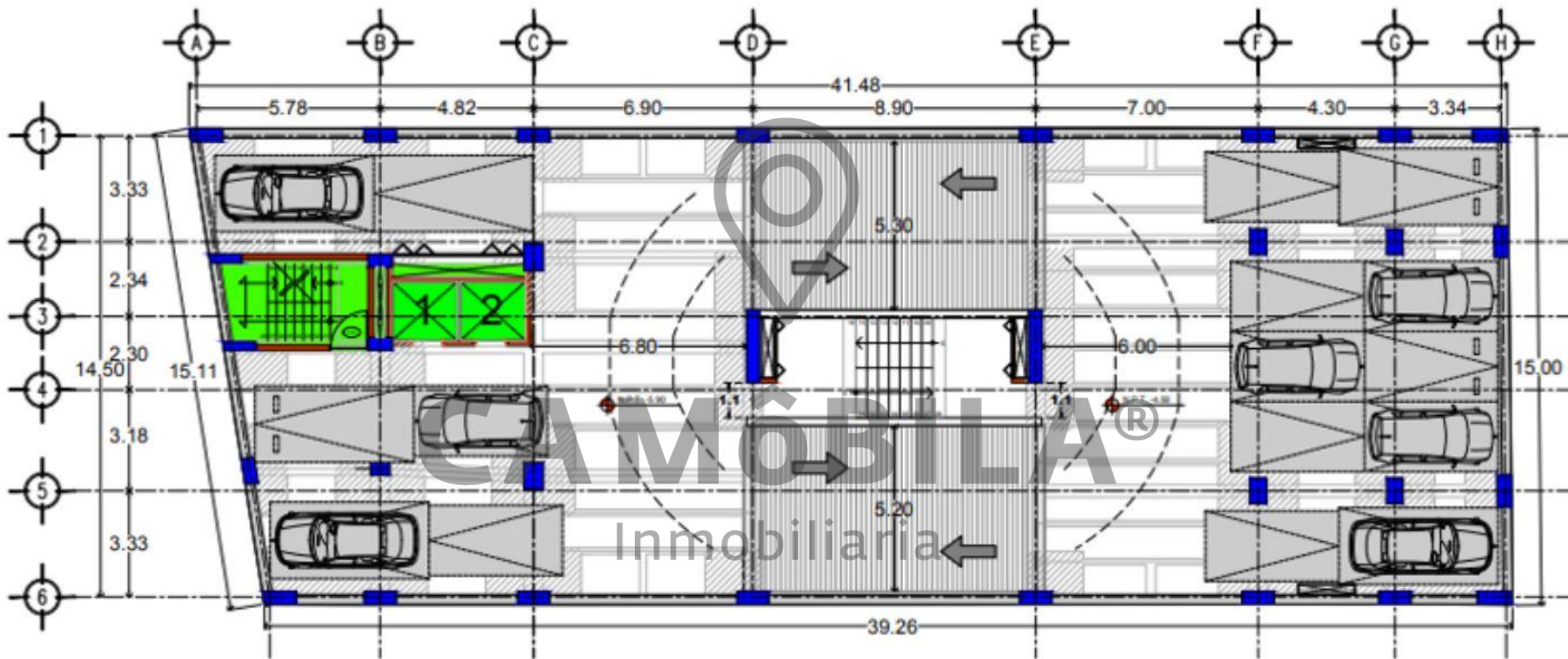
ESTACIONAMIENTO TIPO
