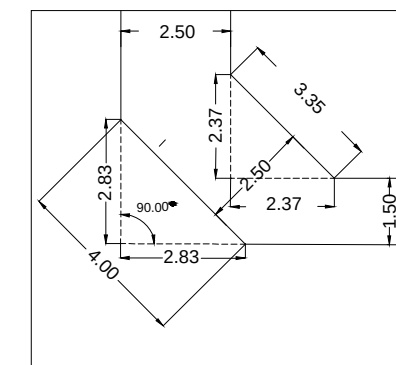
DETALLES DE CHAFLÁN sin escala
