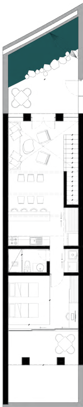
PLANTA BAJA
