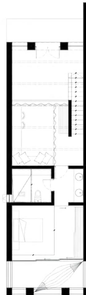
PLANTA ALTA
