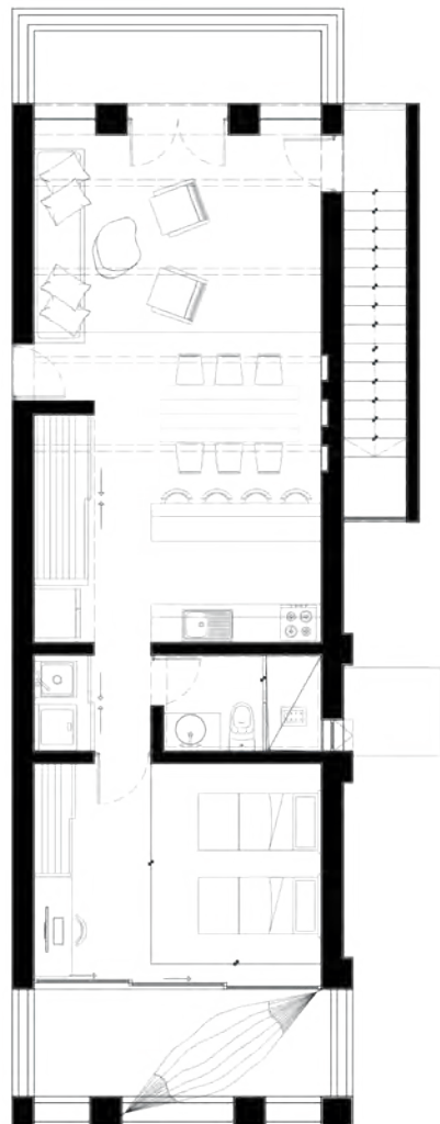
PLANTA BAJA
