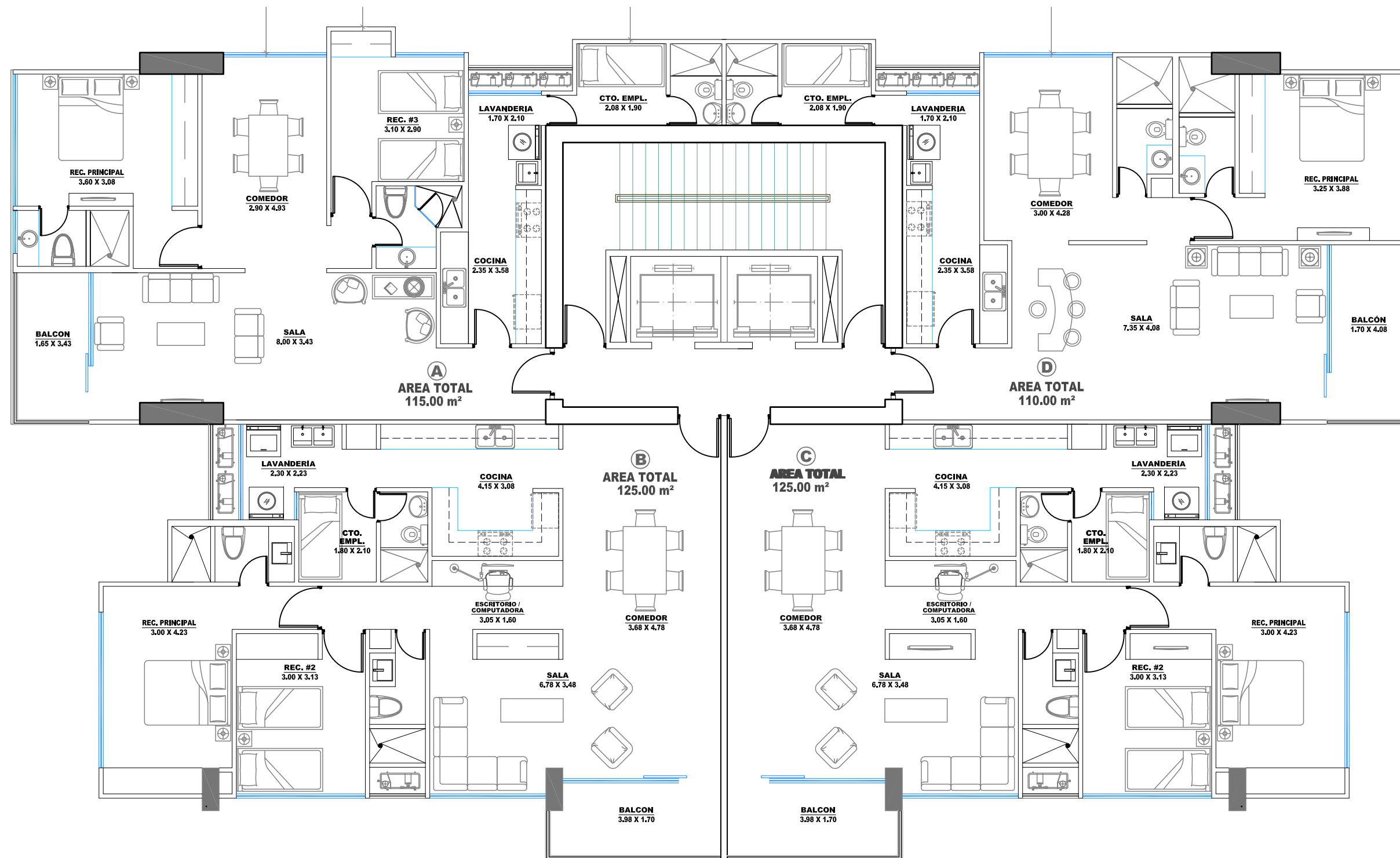
PLANTA DE APARTAMENTOS NIV. 600 @ 2900 ESC.: 1:100
