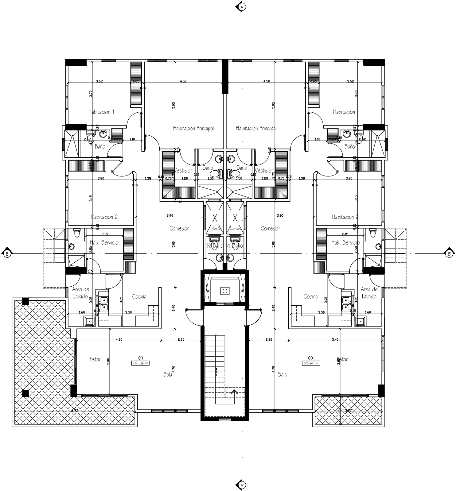
PLANTA ARQUITECTONICA DIMENSIONADA 3er. AL 5to. NIVEL
