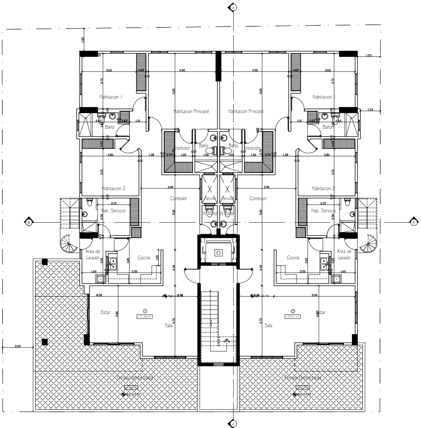
PLANTA ARQUITECTONICA DIMENSIONADA 2do. NIVEL SC. 1:75
