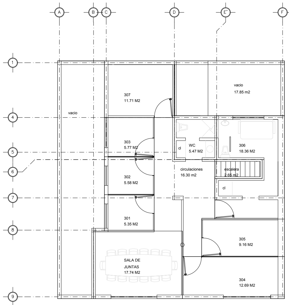
SEGUNDO NIVEL
