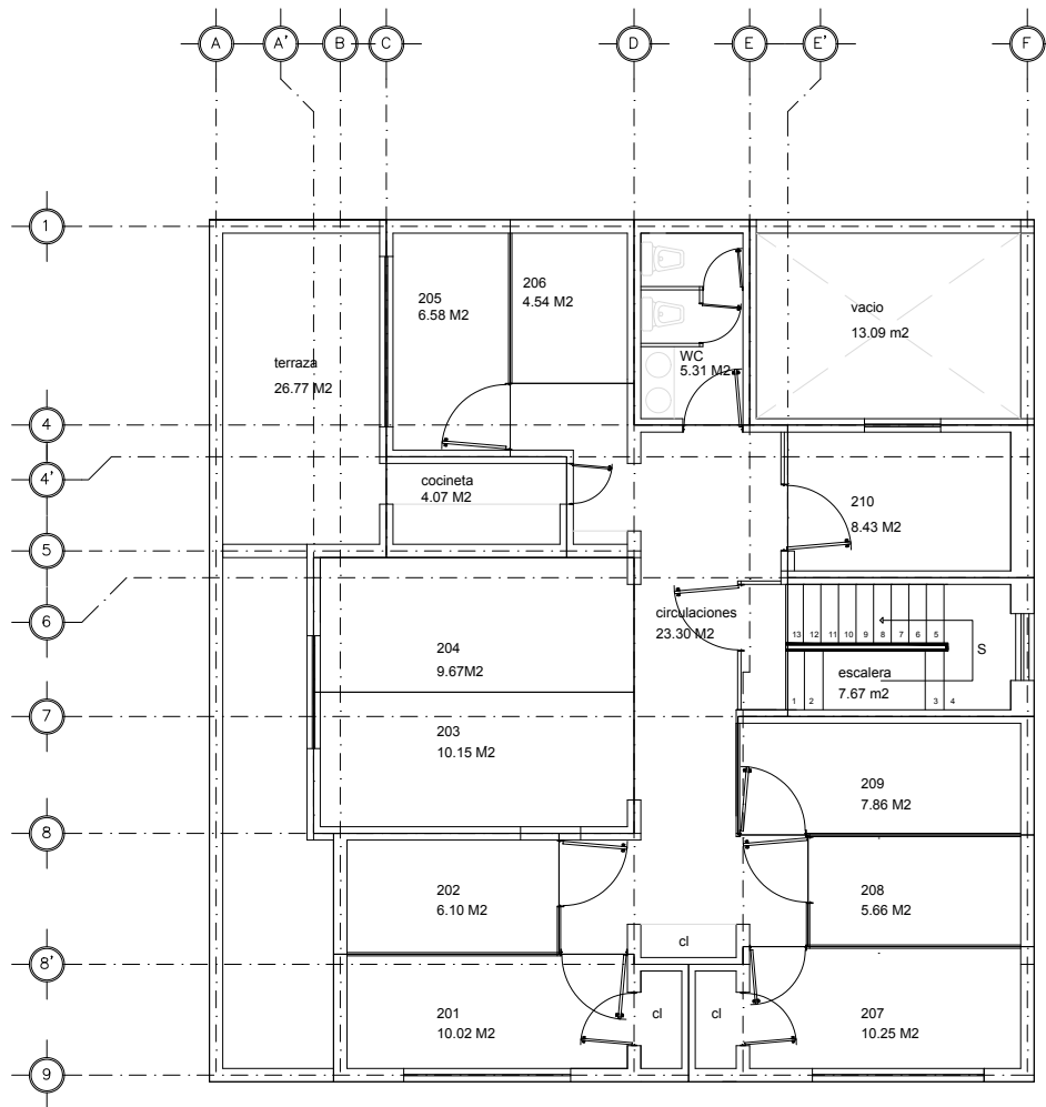
PRIMER NIVEL
