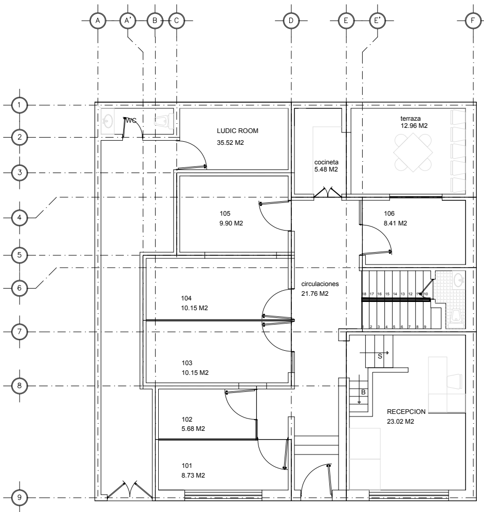
PLANTA BAJA
