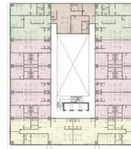
Planta Piso 4 al 16
