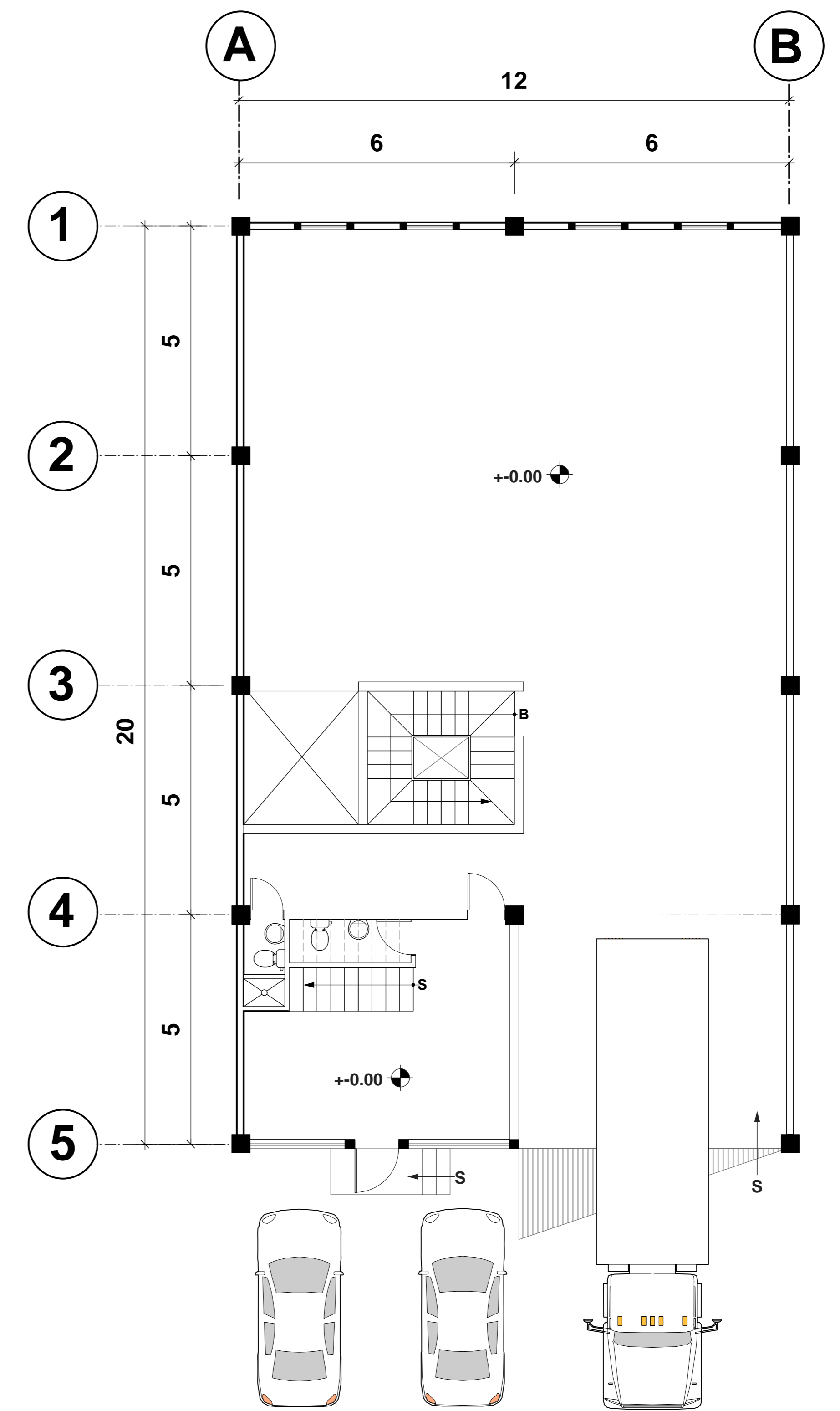
PLANTA TIPICA NIVEL 1 OFIBODEGA
