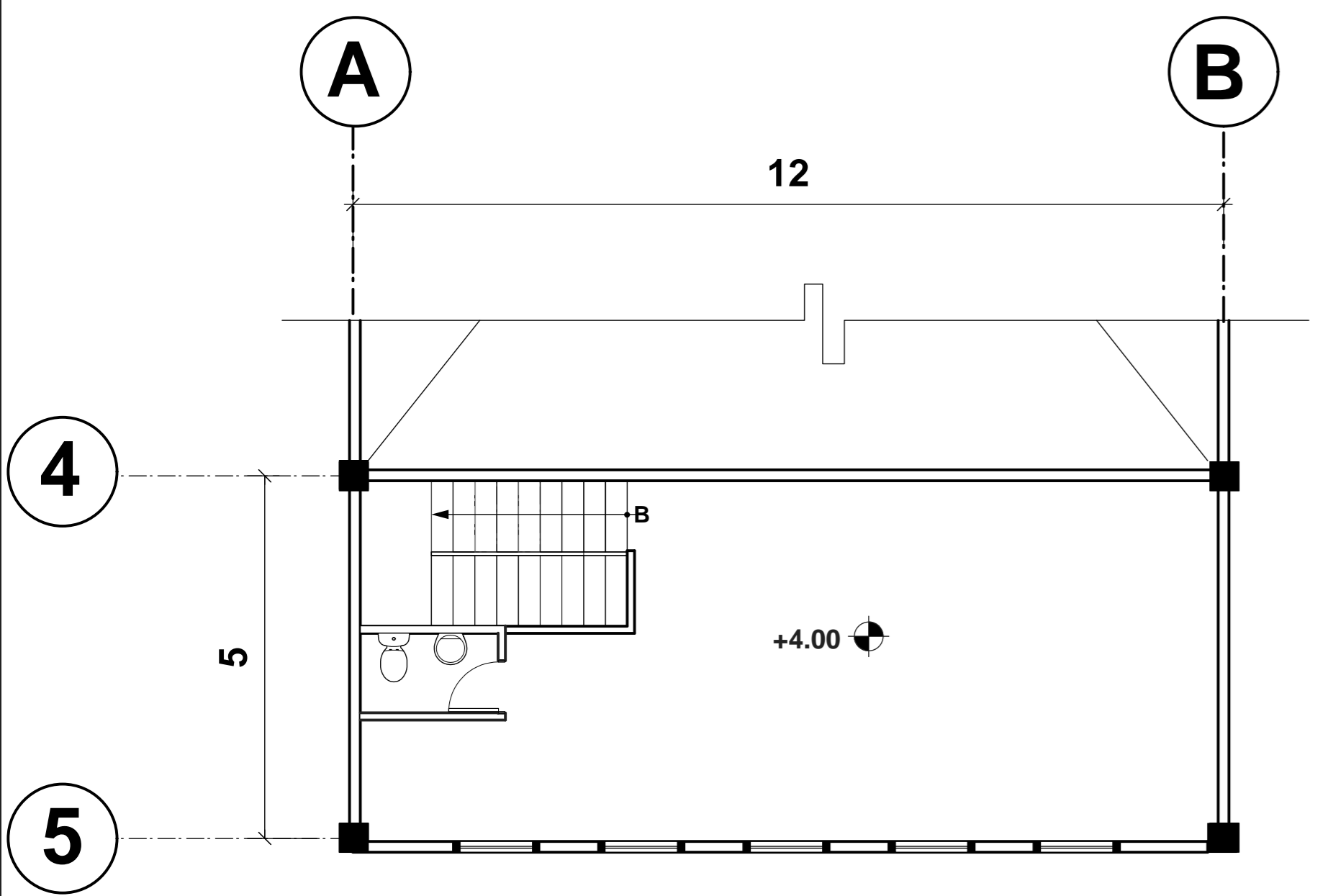
PLANTA TIPICA MEZANINE OFIBODEGA
