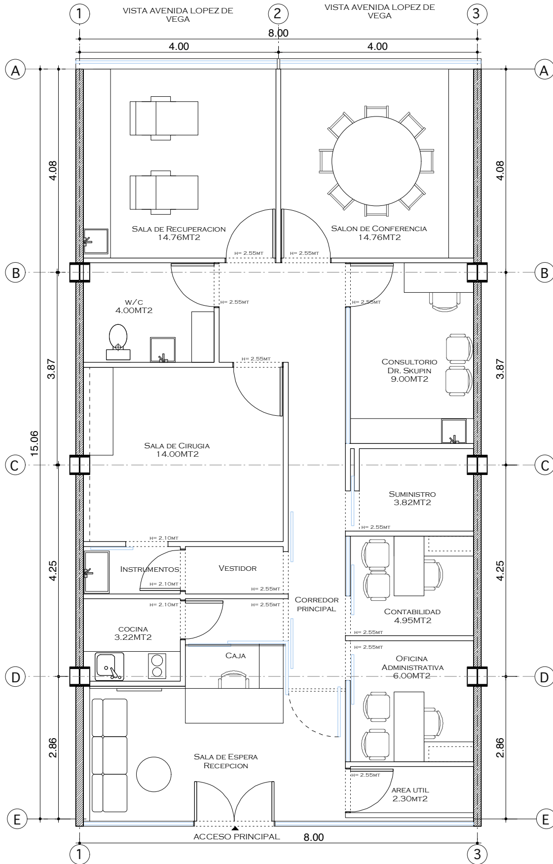
1 PLANTA ARQUITECTONICA Scale: 1:75
