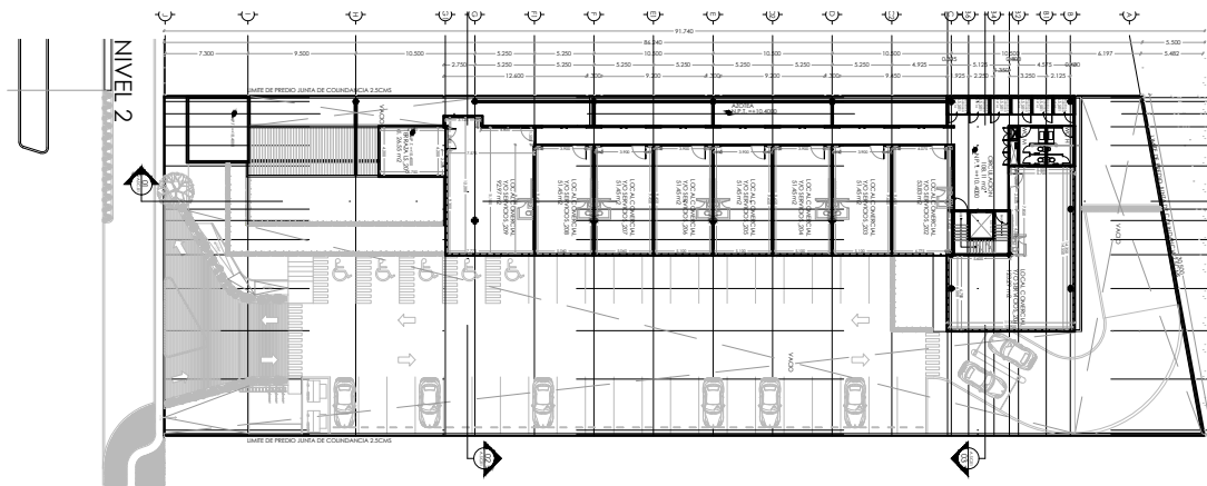
Detalle de Condominio / Ubicación de la Unidad Condominial Sin Escala
