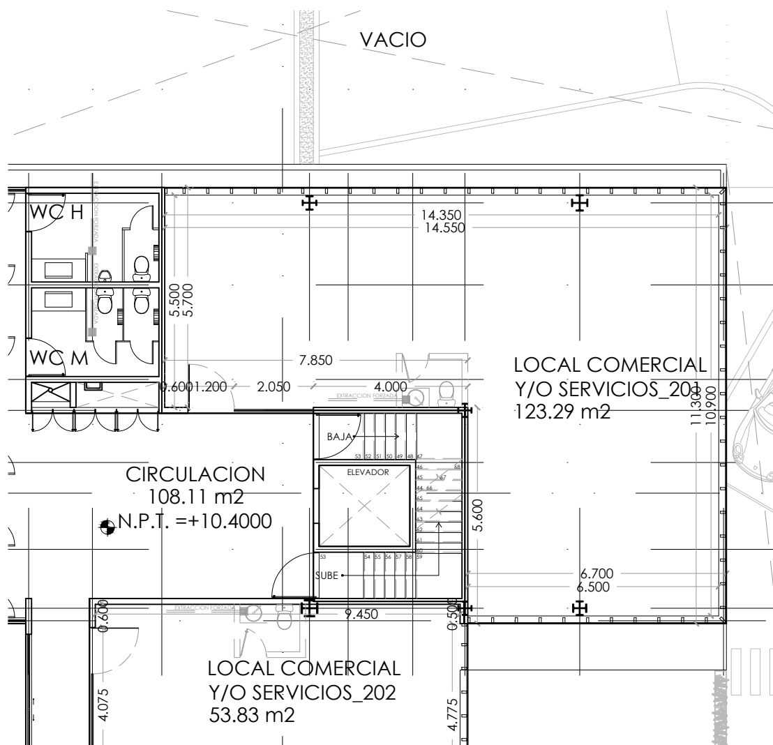
Detalle de Unidad Condominial Sin Escala
