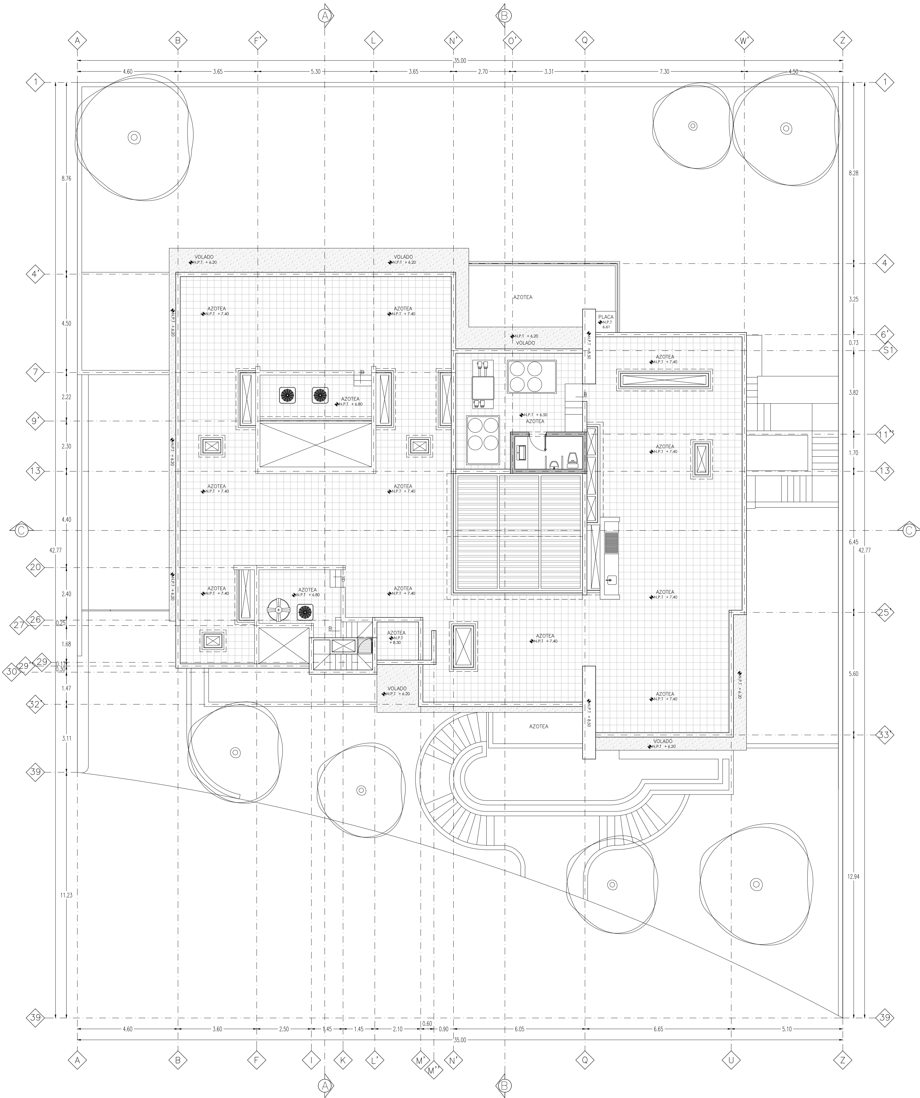
PLANTA AZOTEAS ESC 1:100
