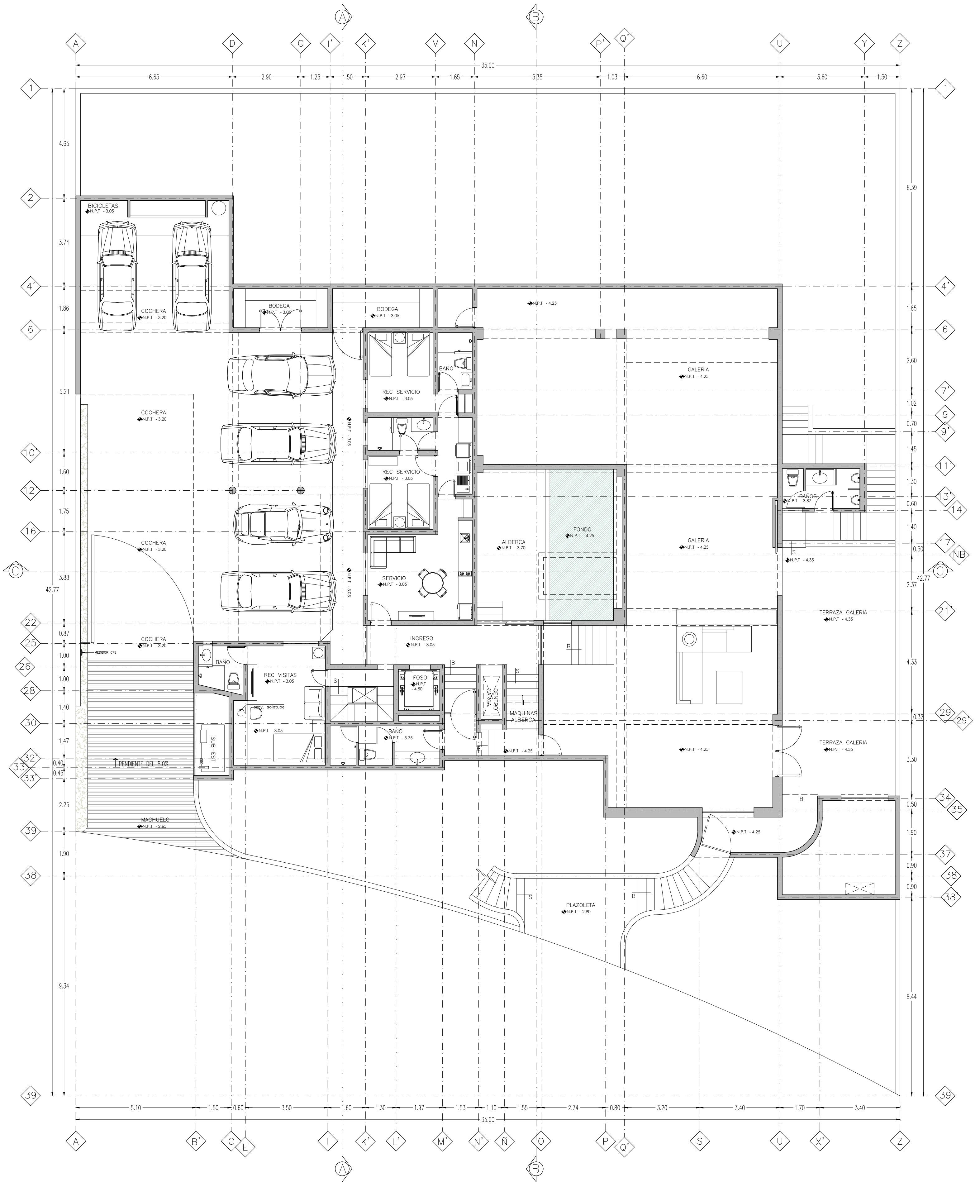
PLANTA SOTANO ARQUITECTONICA ESC 1:100
