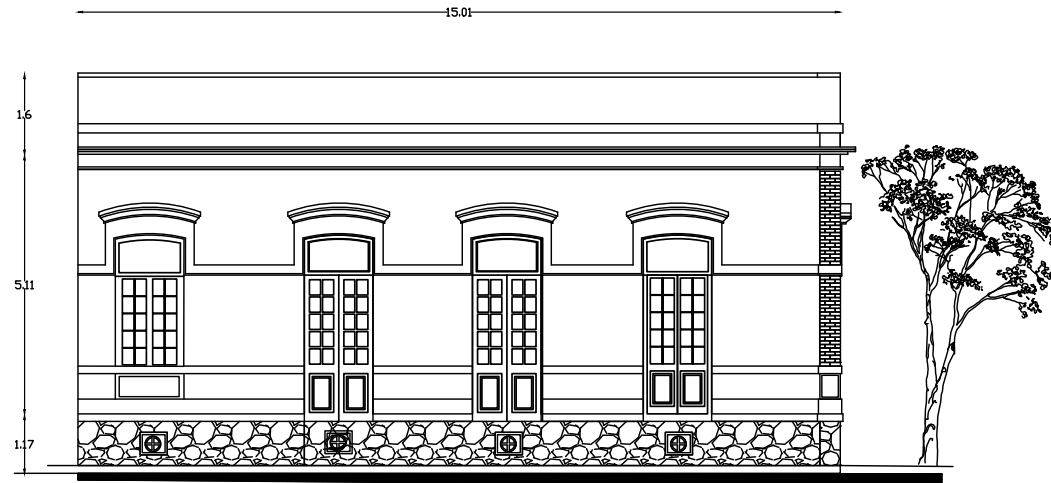
FACHADA SUR
