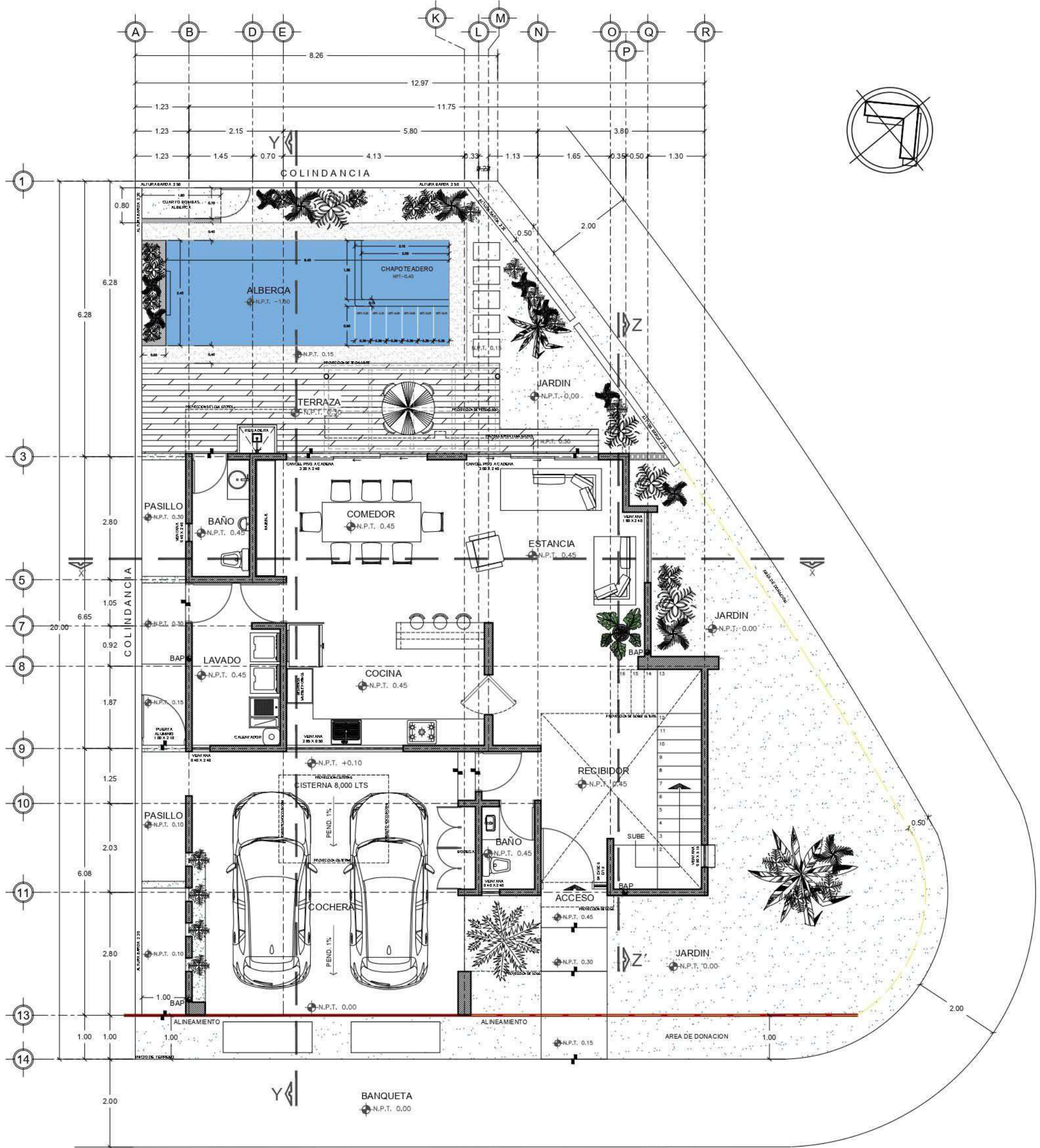
PLANTA BAJA (120.98 m2)
