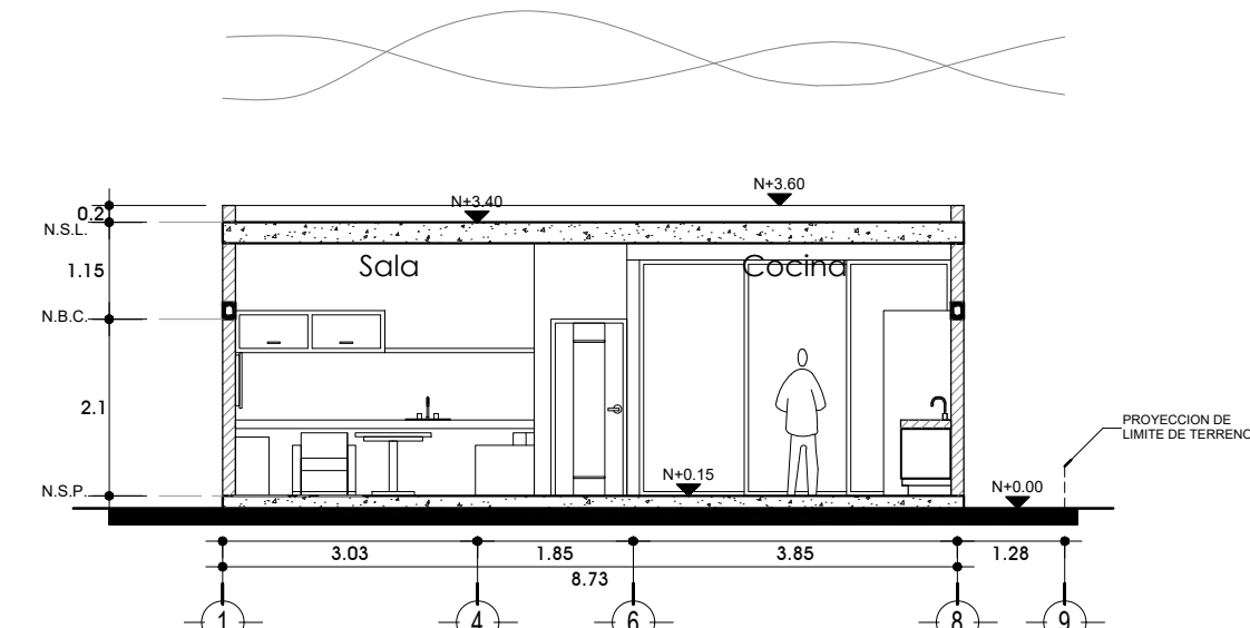
Corte Arquitectónico X-X'
