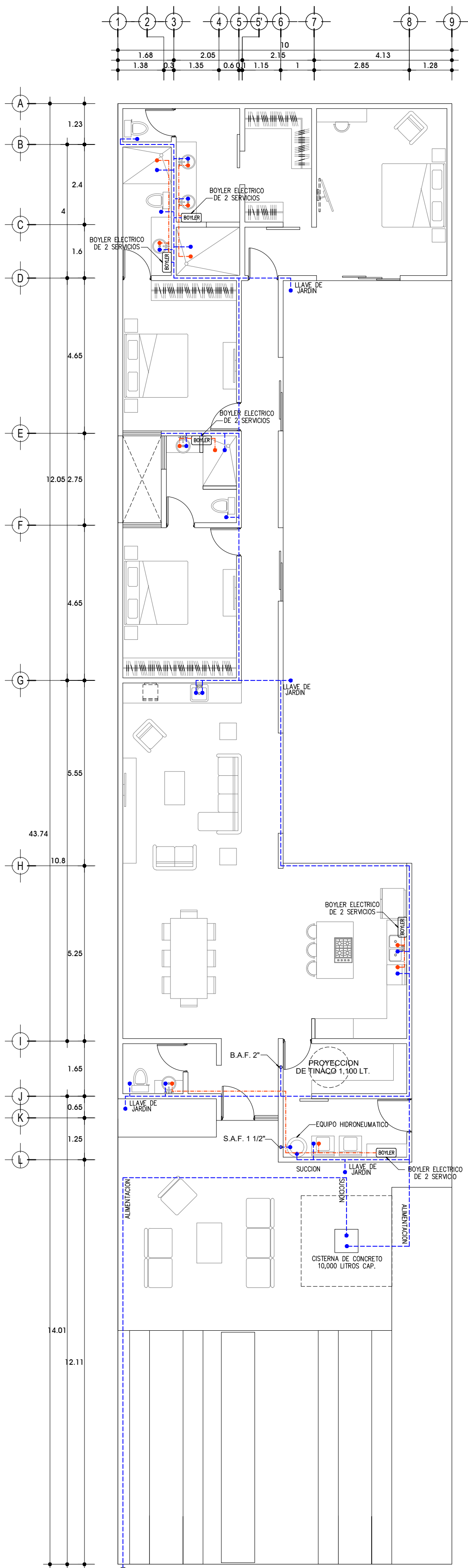
Planta Hidraulica
