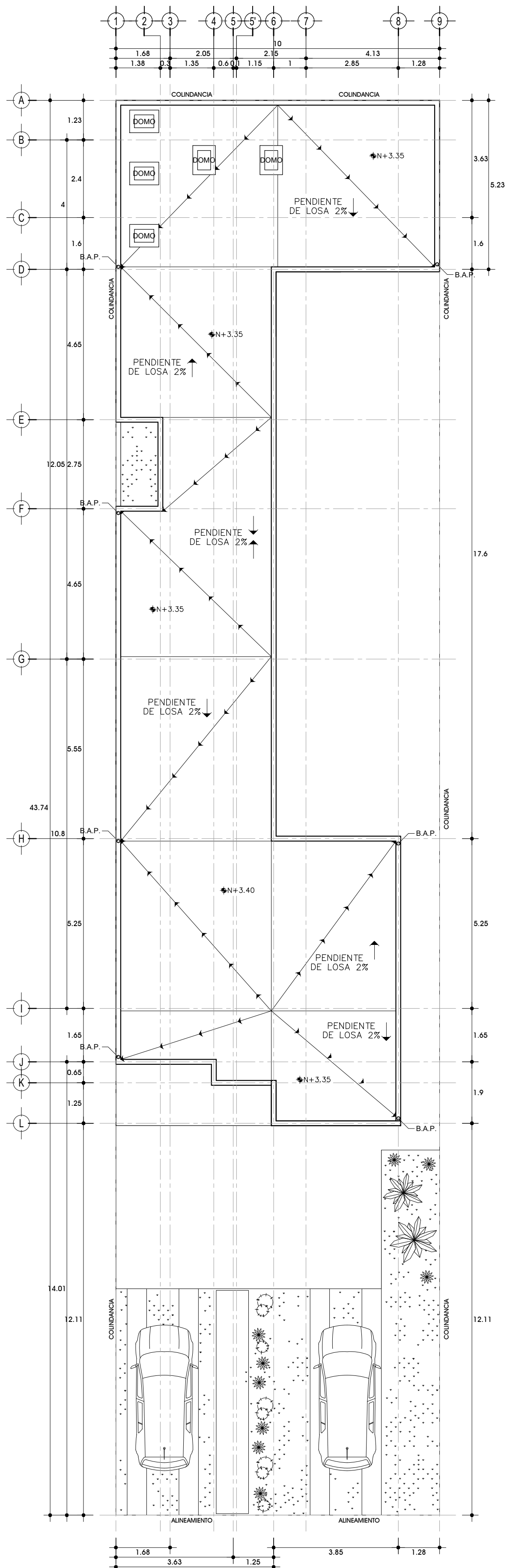
Planta de Azotea
