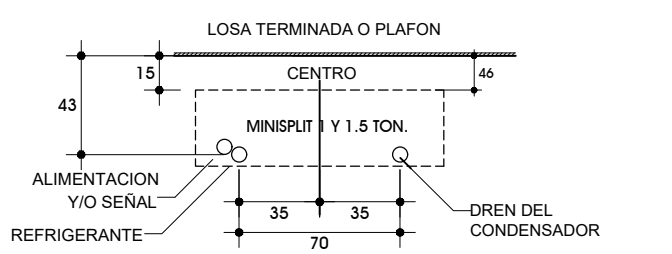
detalle de colocacion minisplit
