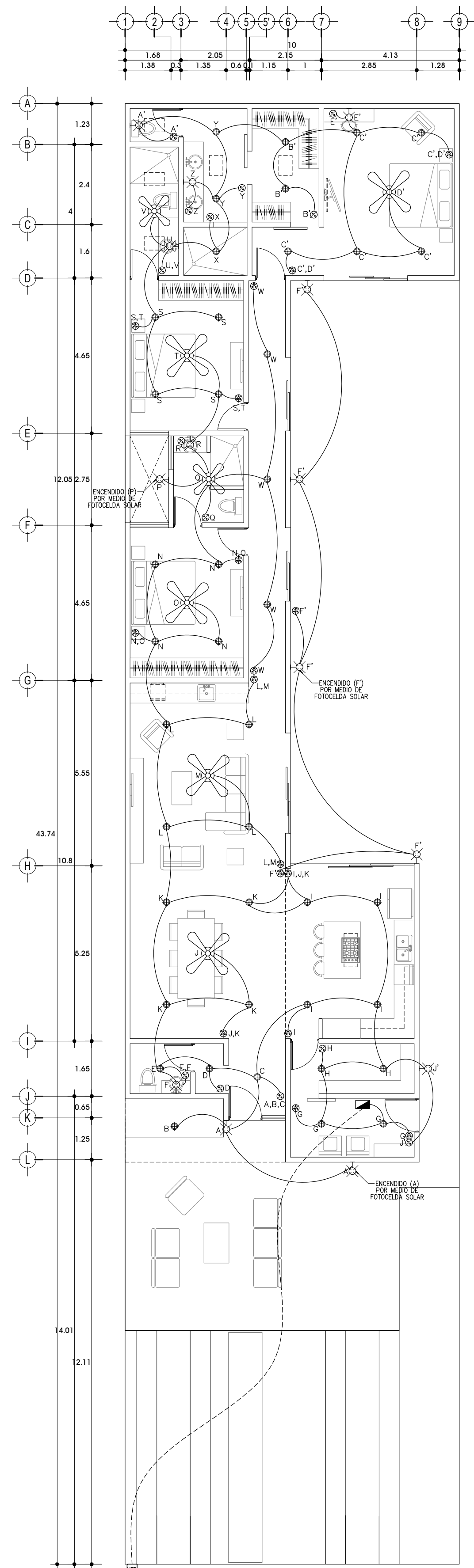
Planta Electrica de Iluminacion
