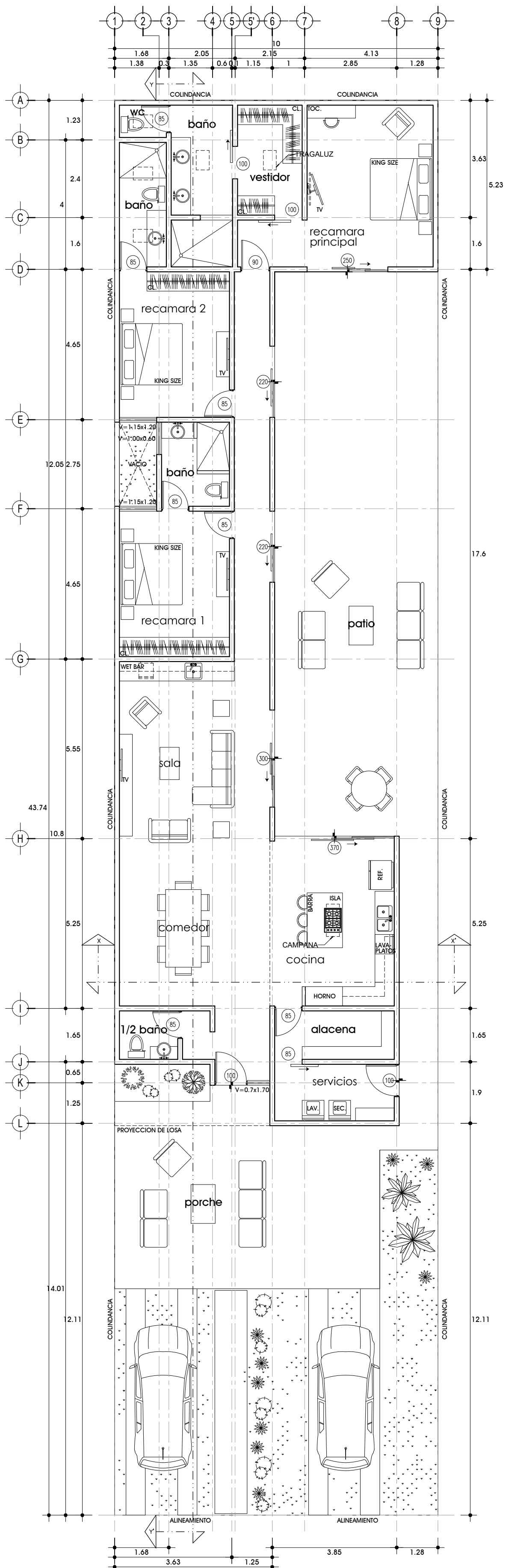
Planta Arquitectónica Área: 214.76 M2
