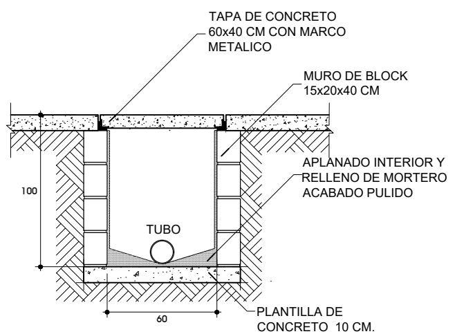
registro sanitario tipo
