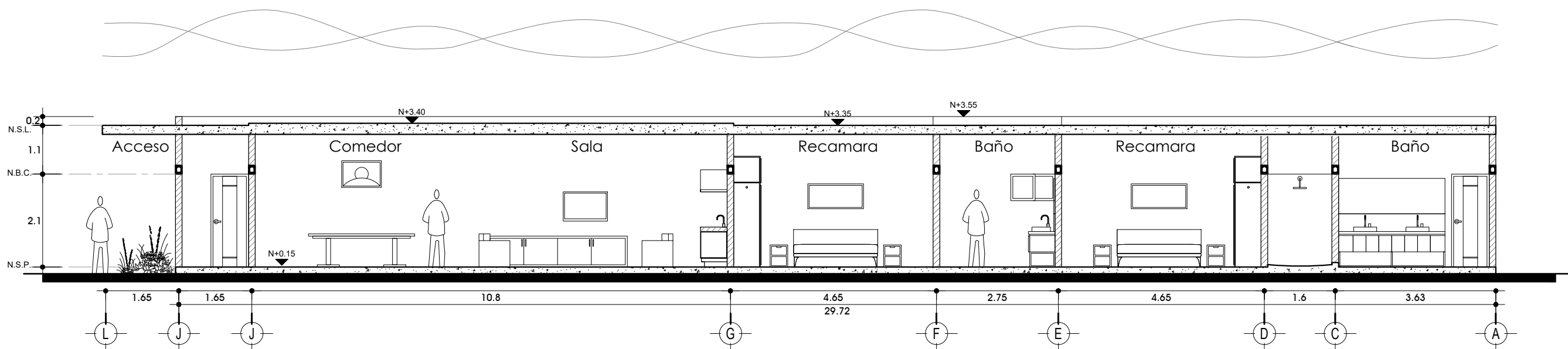
Corte Arquitectónico Y-Y'
