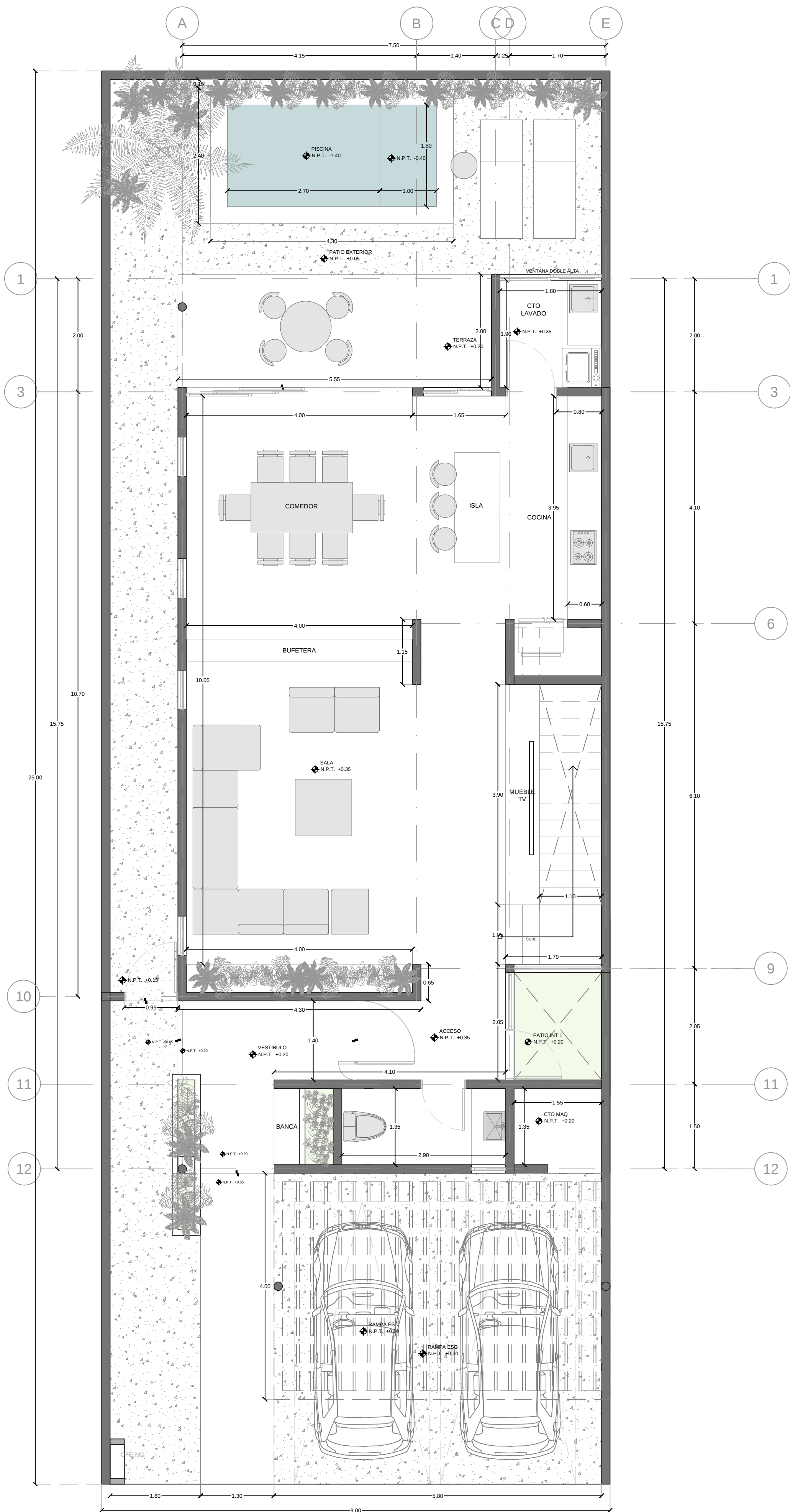
PLANTA BAJA
