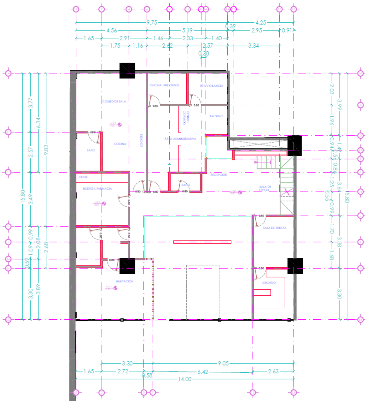
PLANOS PLANTA ALTA
