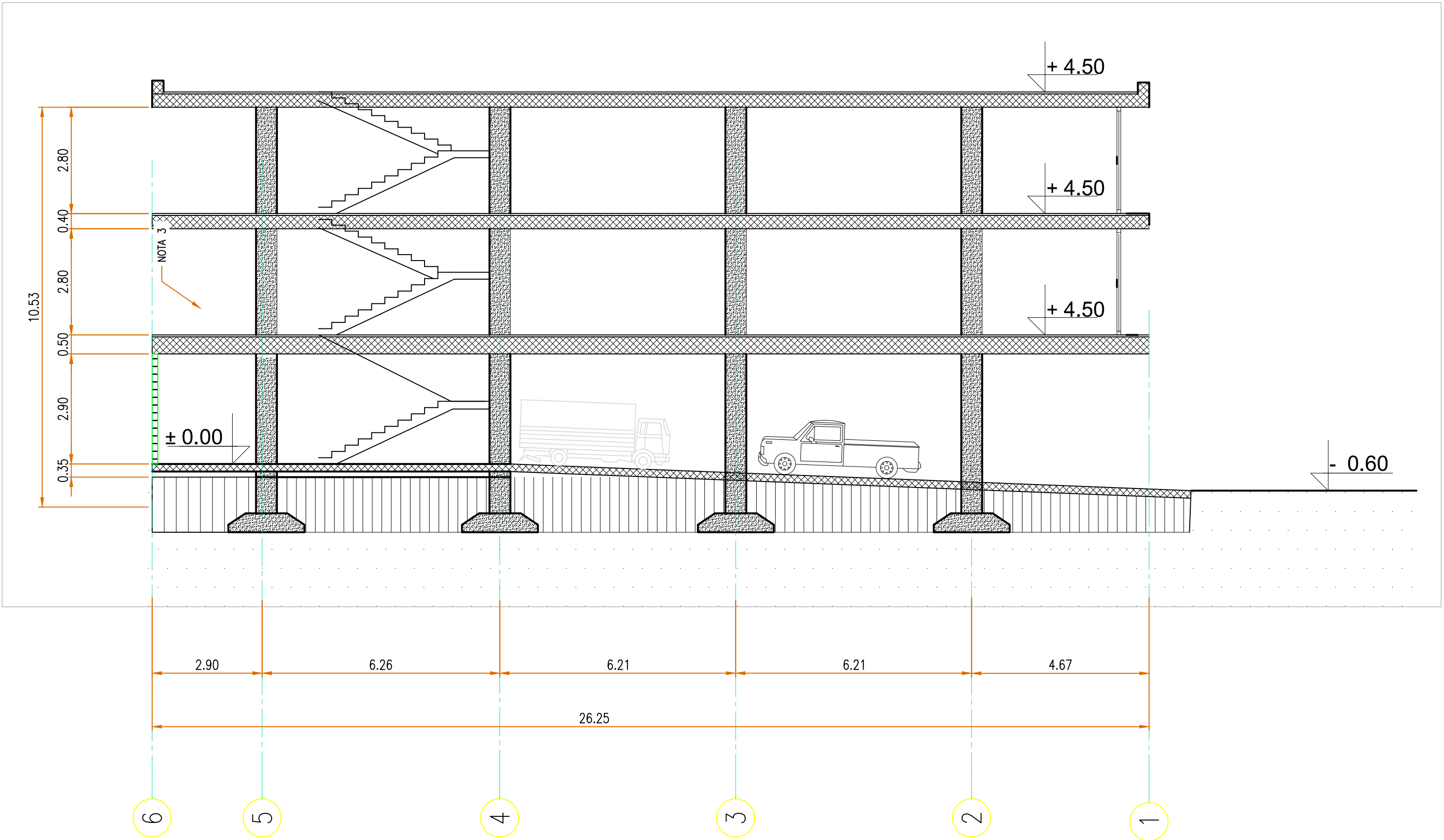
Corte Vista 1 - 1 ESCALA: 1/10
