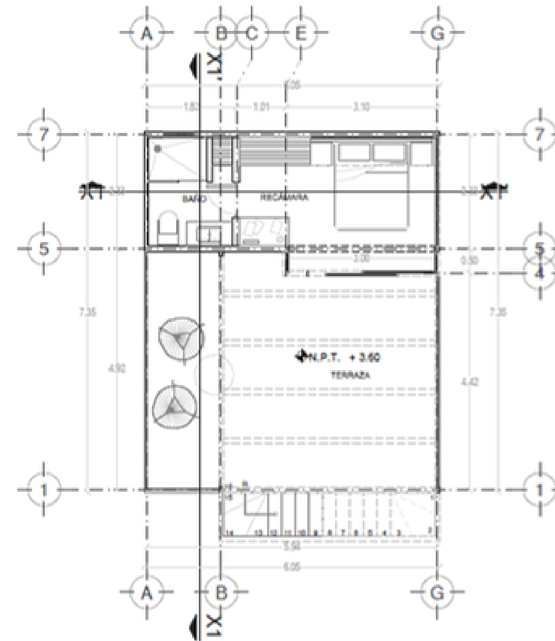
PLANTA ALTA ESCALA 1:75
