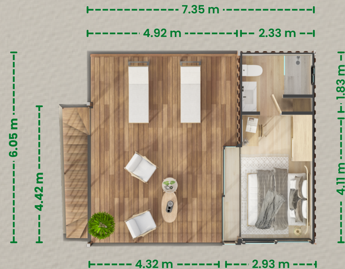
Planta alta
