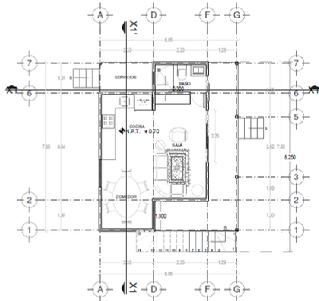
PLANTA BAJA ESCALA 1:75
