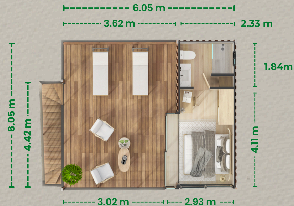
Planta Alta
