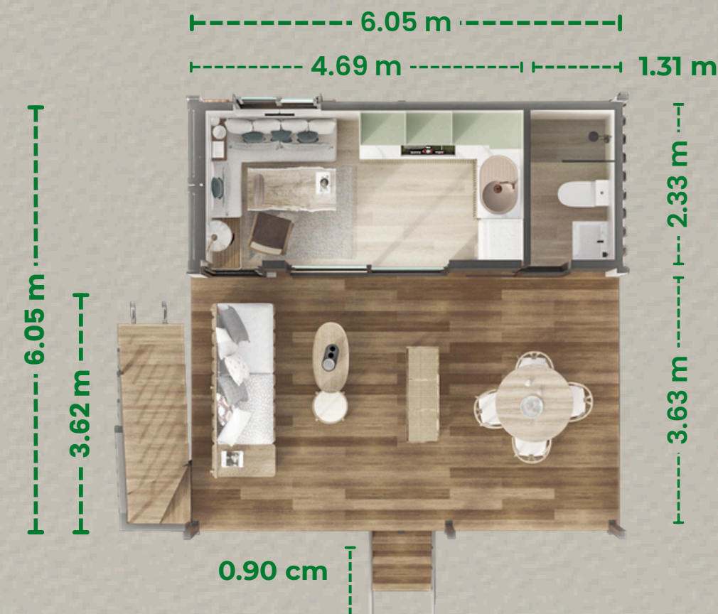
Planta baja
