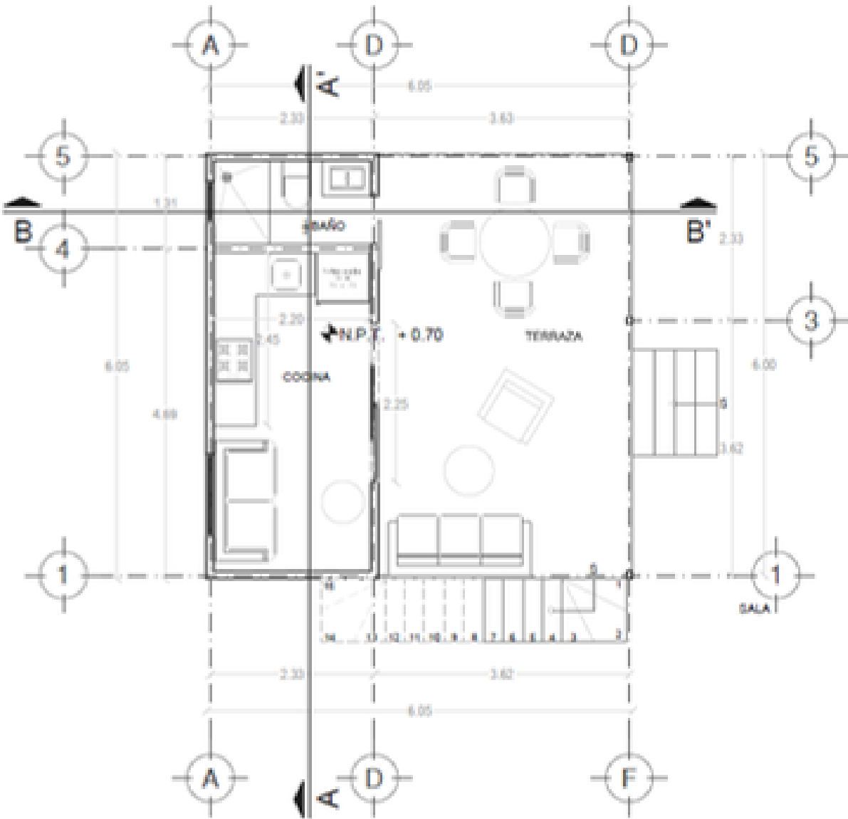
PLANTA BAJA ESCALA 1:75
