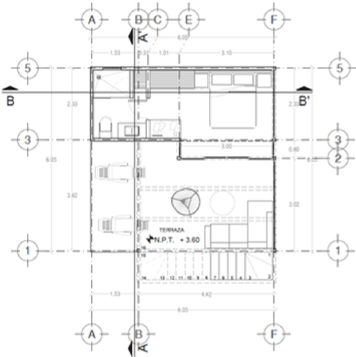
PLANTA ALTA ESCALA 1:75
