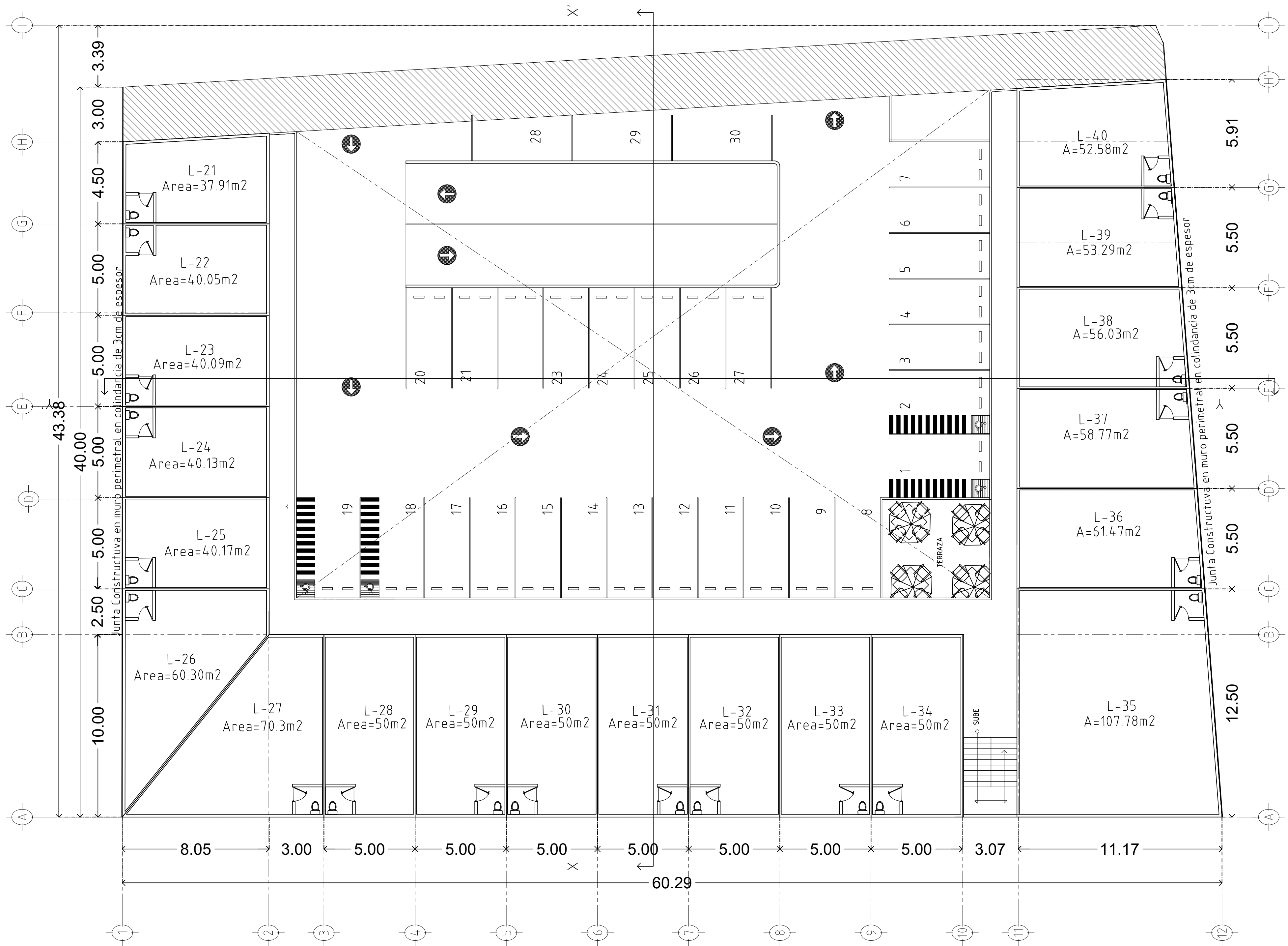
PLANTA ARQUITECTONICA PLANTA ALTA
