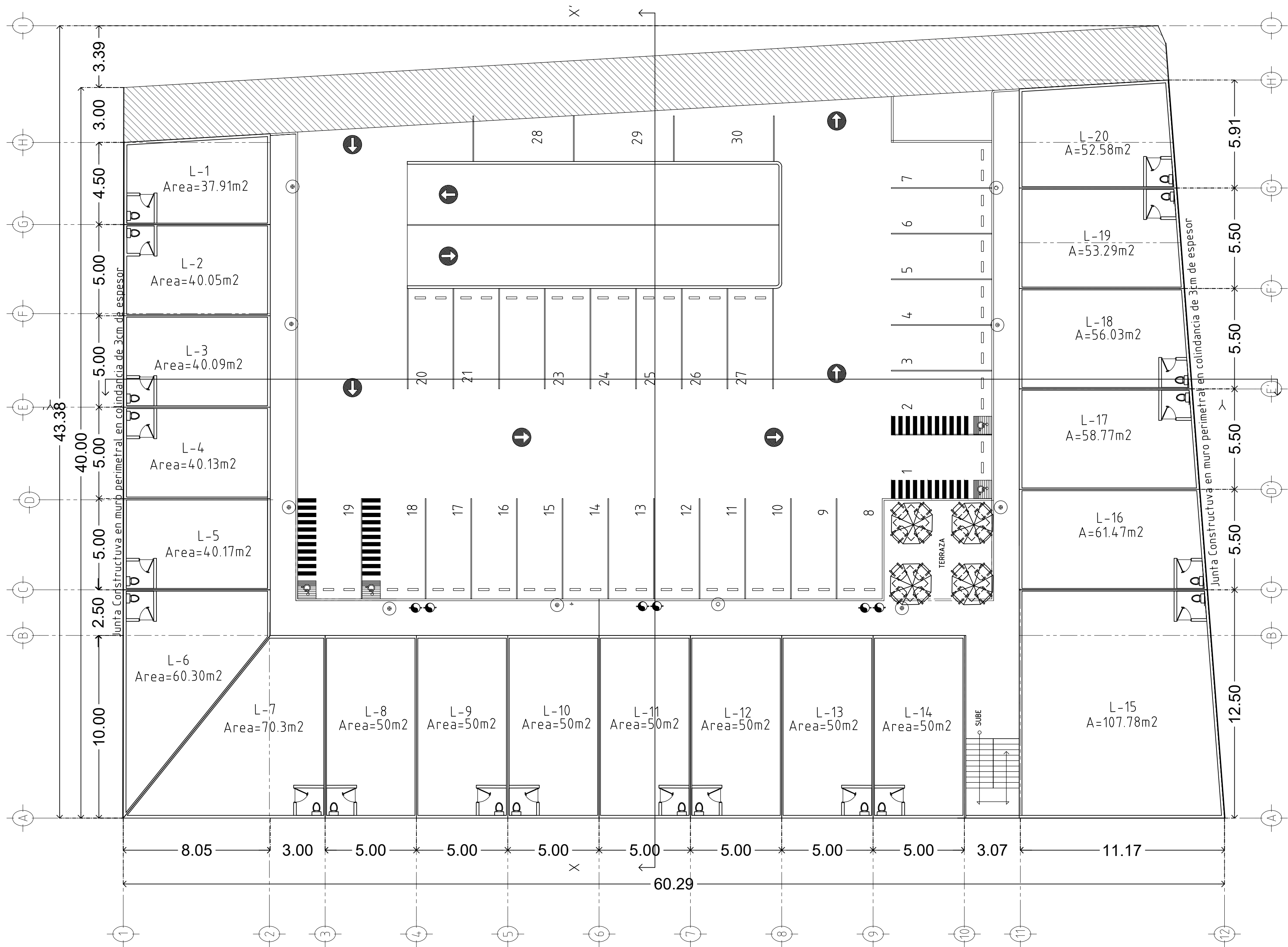
PLANTA ARQUITECTONICA PLANTA BAJA
