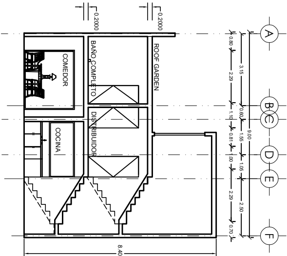
CORTE TRANSVERSAL
