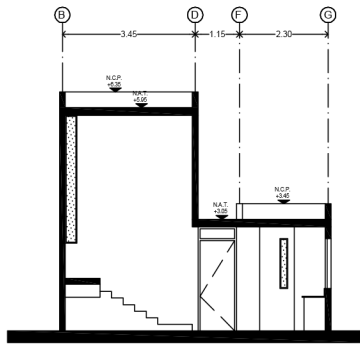
SECCIÓN X1
