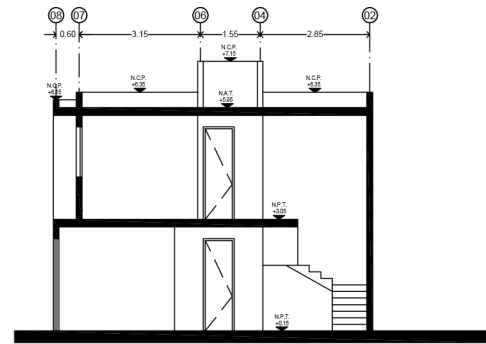
SECCIÓN Y1
