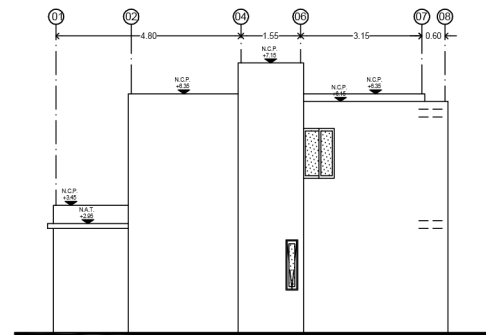
FACHADA LATERAL
