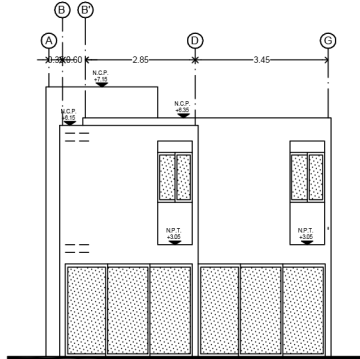
FACHADA TRASERA
