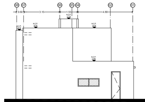
FACHADA LATERAL
