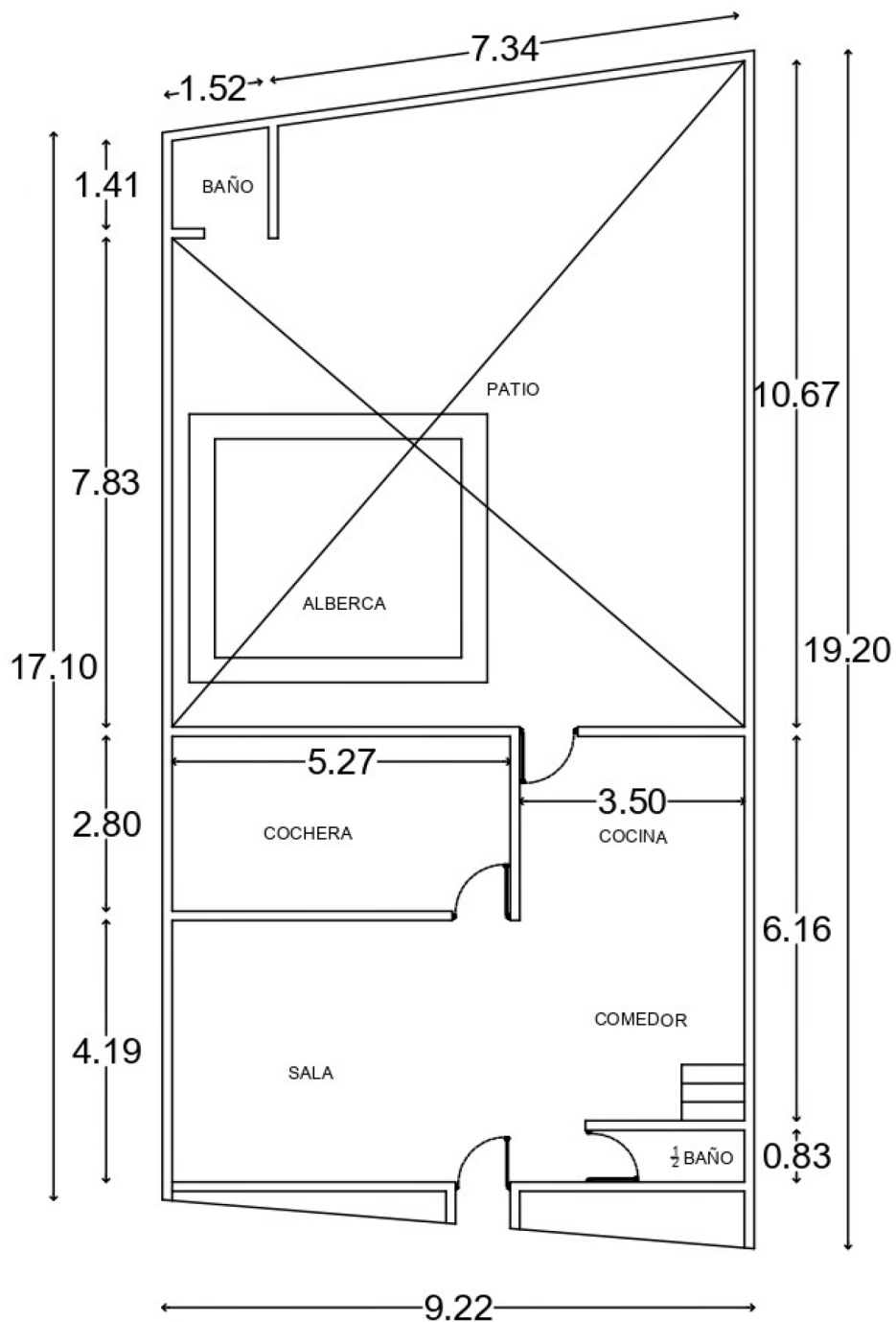
PLANTA BAJA
