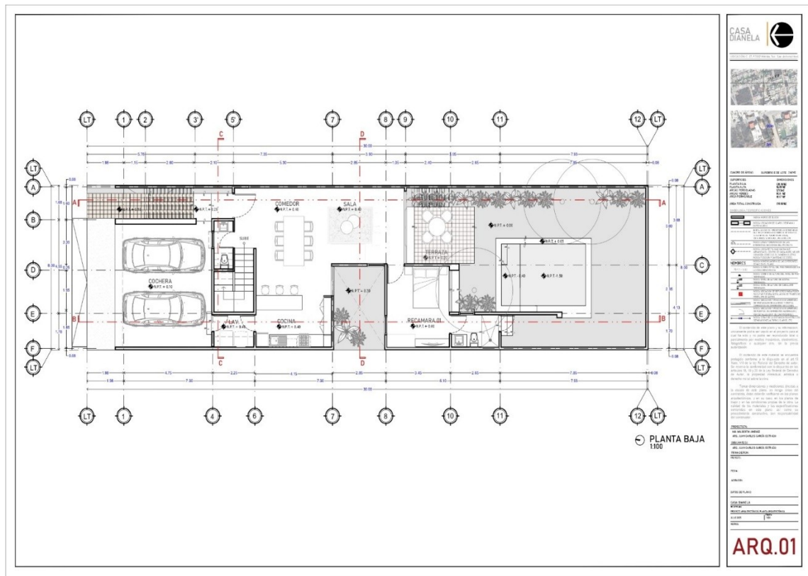
PLANTA ARQUITECTONICA BAJA
