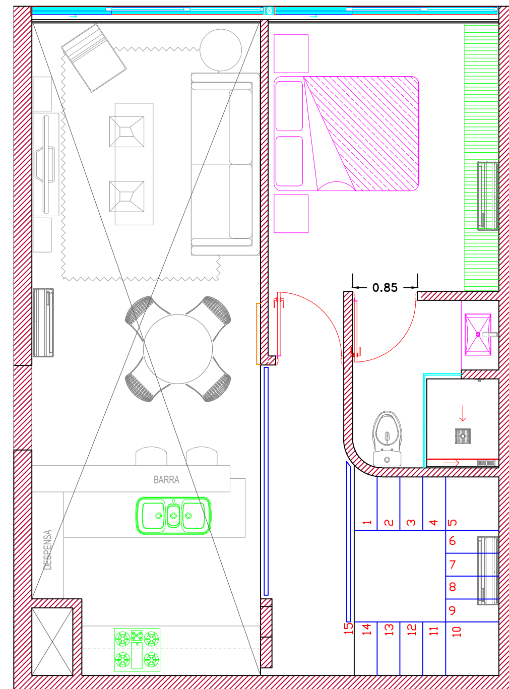
PLANTA ARQUITECTÓNICA ALTA
