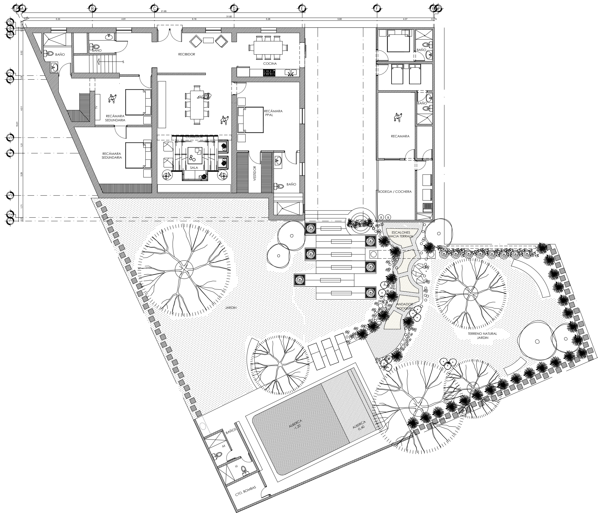
PLANTA ARQUITECTÓNICA PLANTA BAJA
