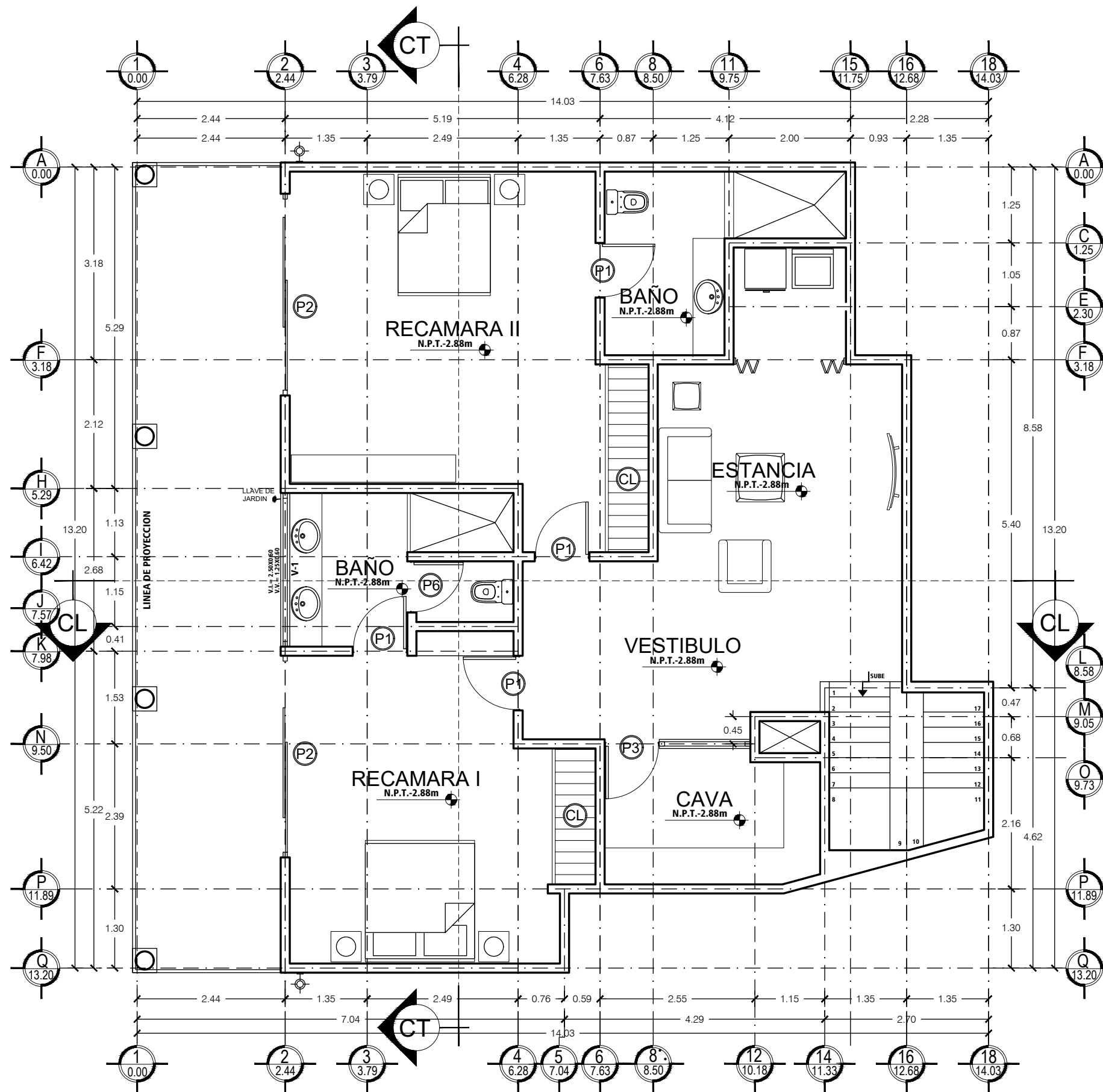
PLANTA ARQUITECTÓNICA Nivel 1 Sup. Const.: 131.41m2. Terraza: 32.54m2
