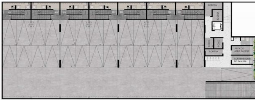
Planta Estacionamiento
