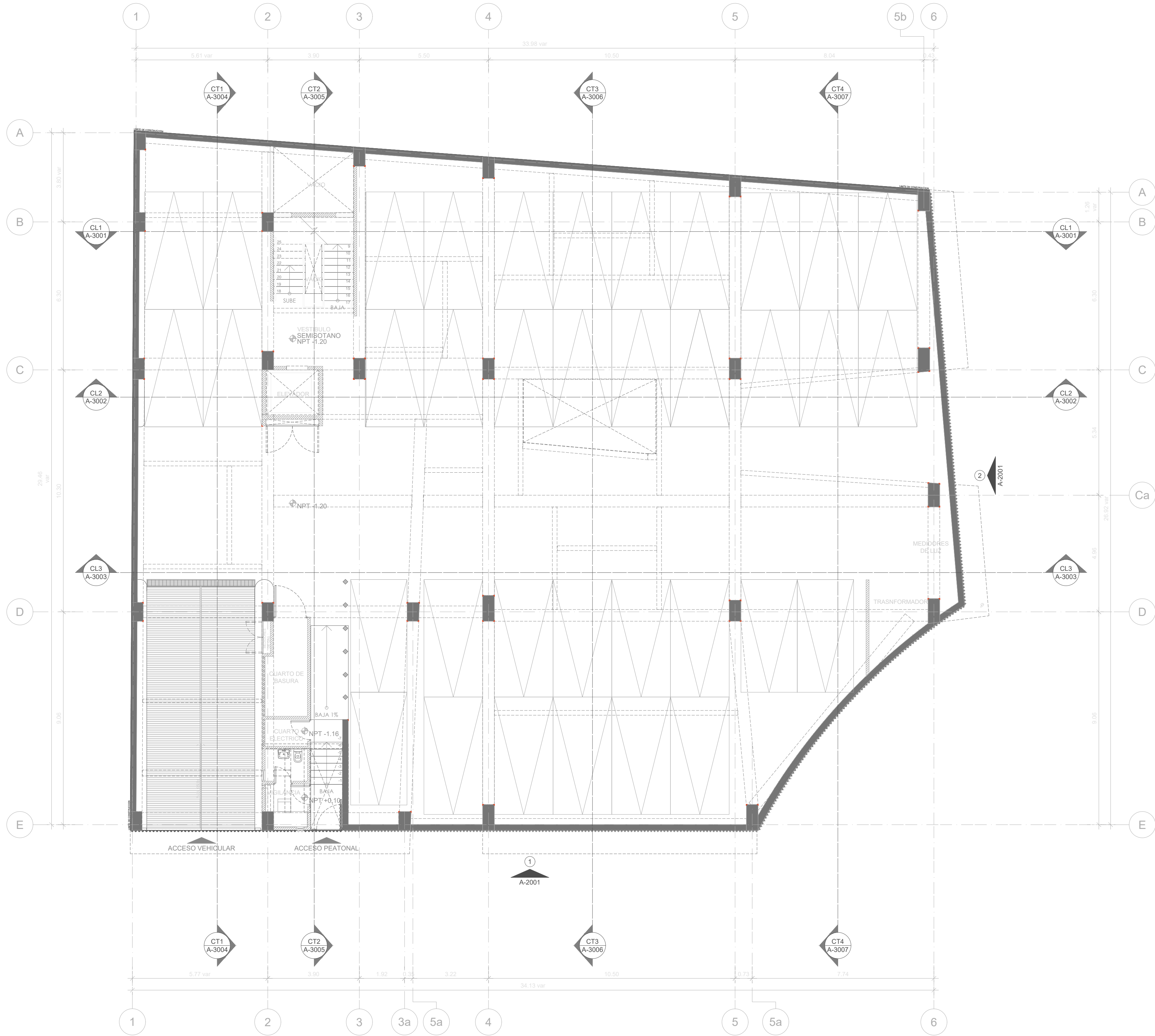
1 SEMISÓTANO 1:100
