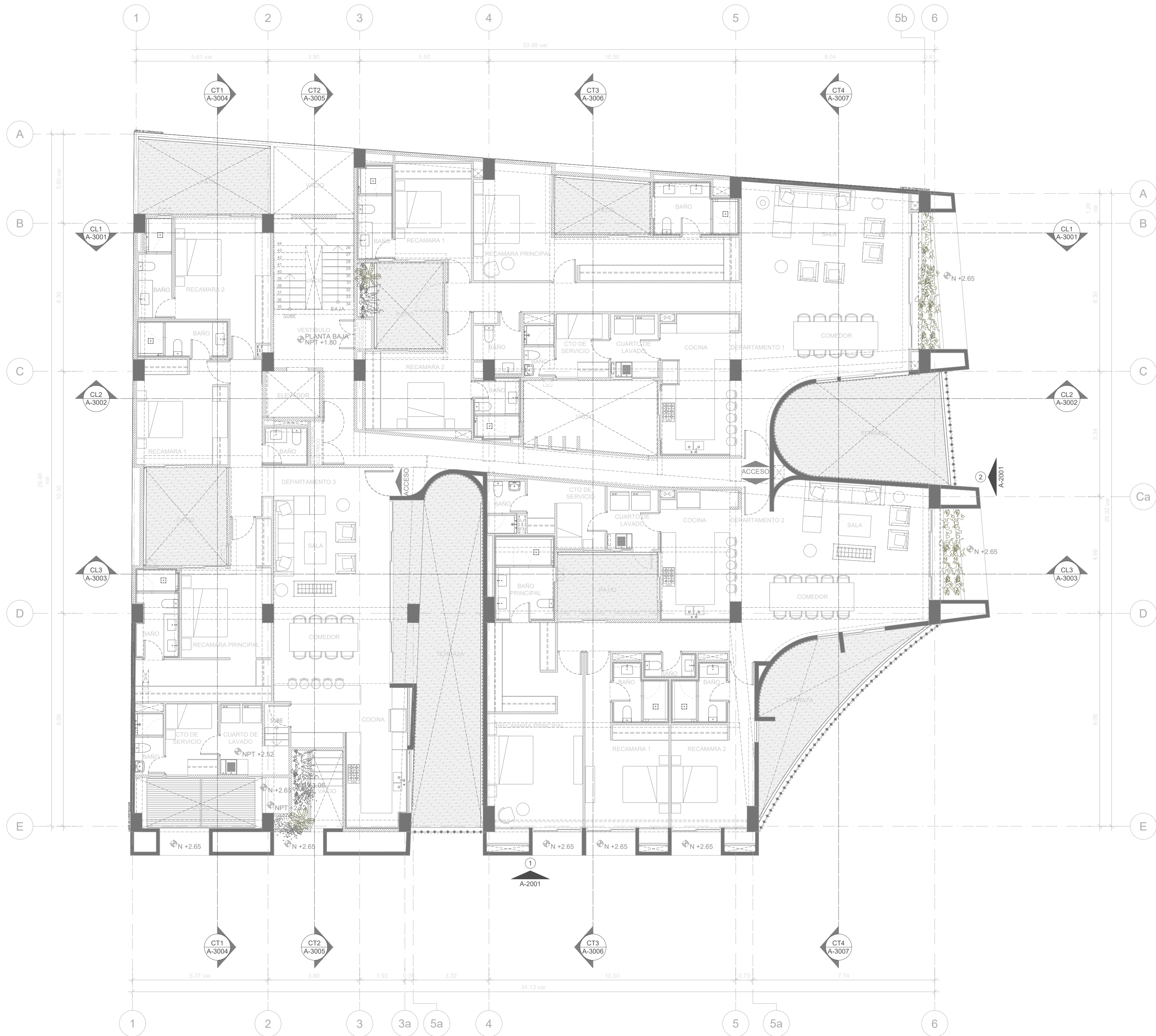
1 PLANTA BAJA 1:100
