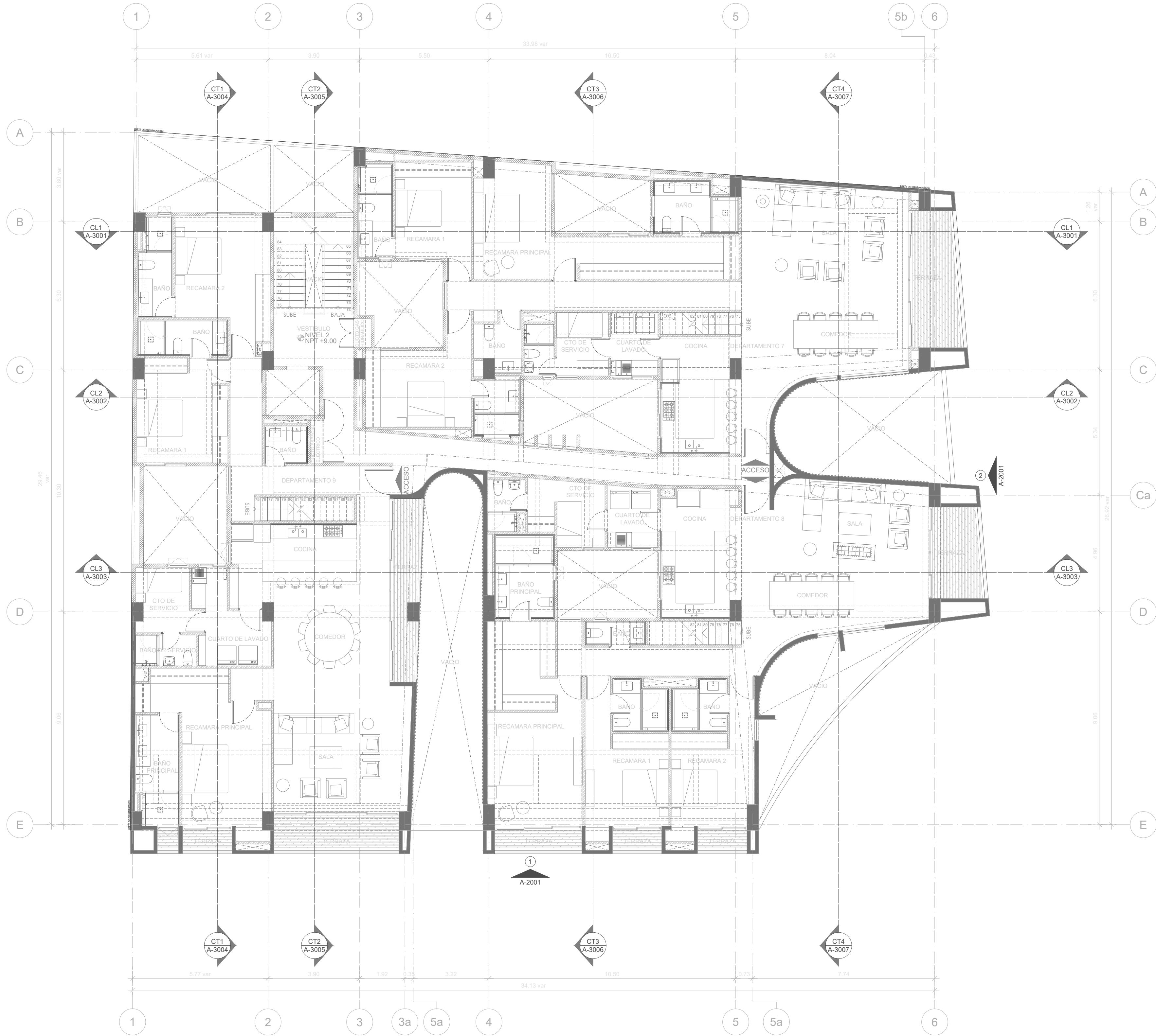
1 NIVEL 2 1:100
