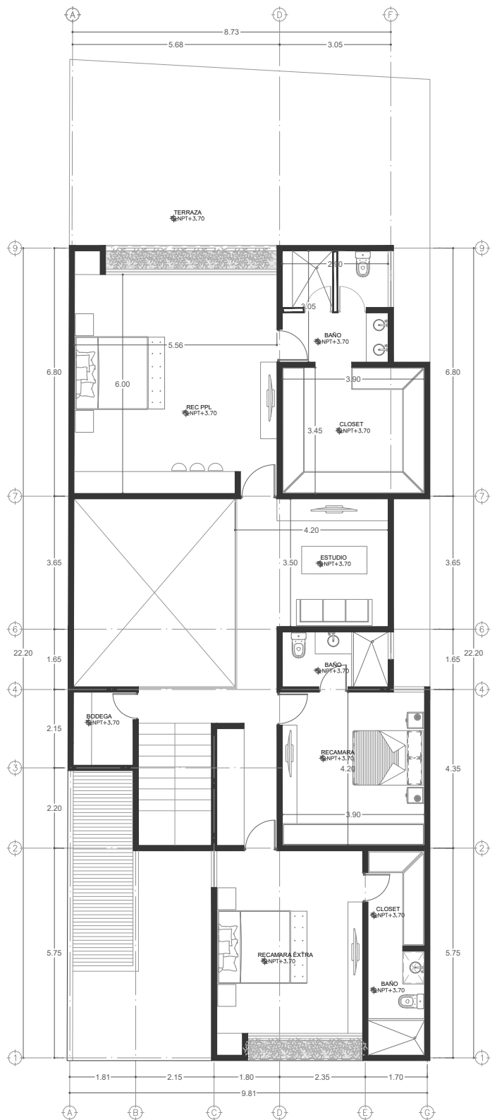
PLANTA ALTA
