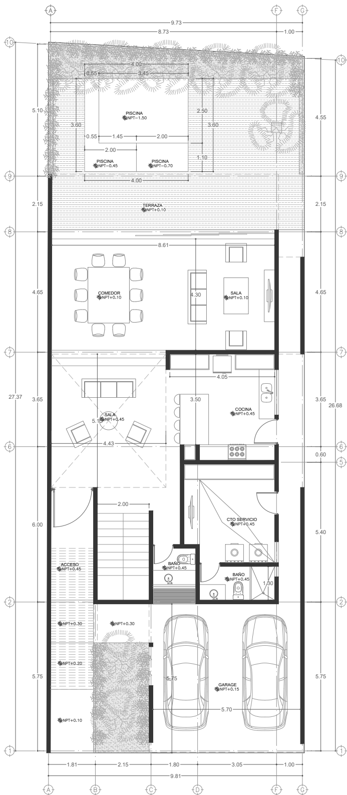
PLANTA BAJA
