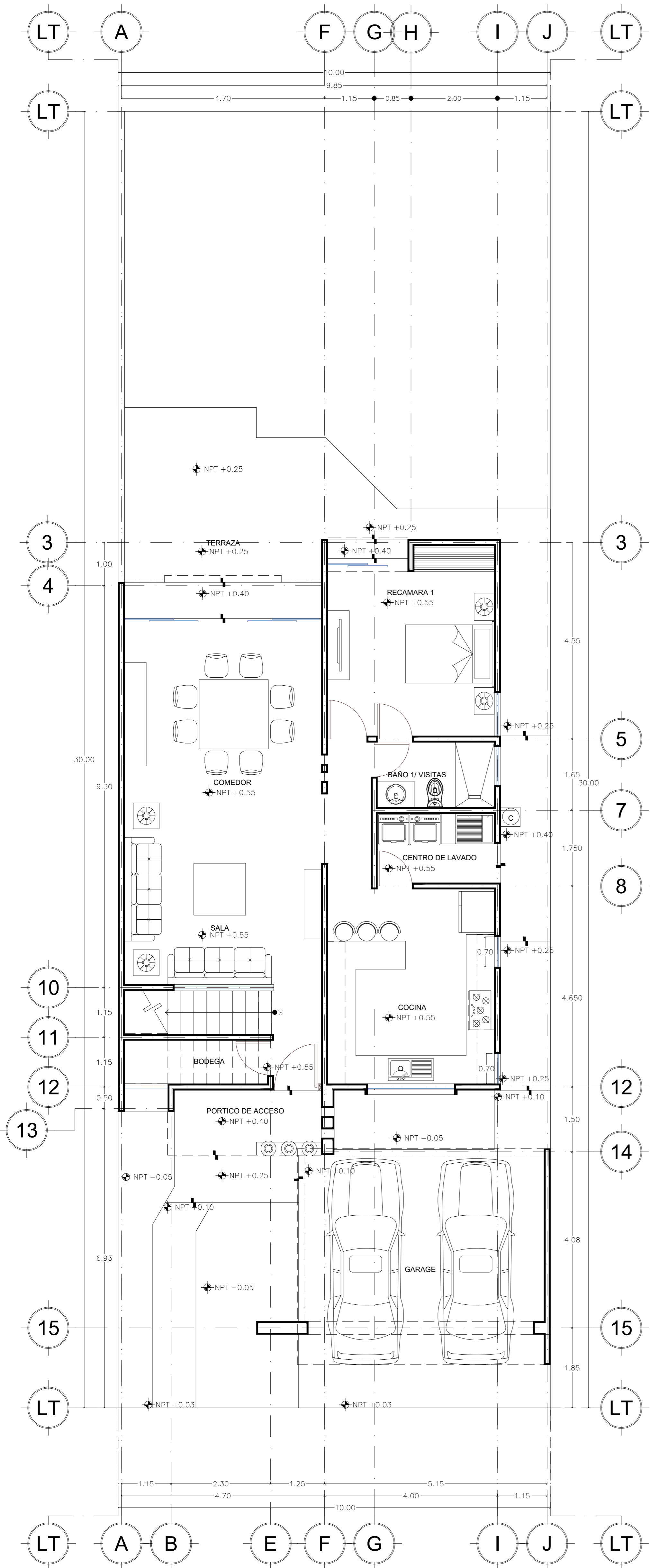
PLANTA BAJA
