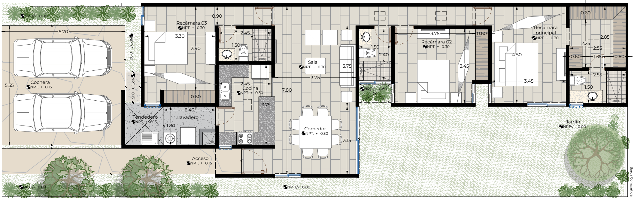
PLANTA BAJA
