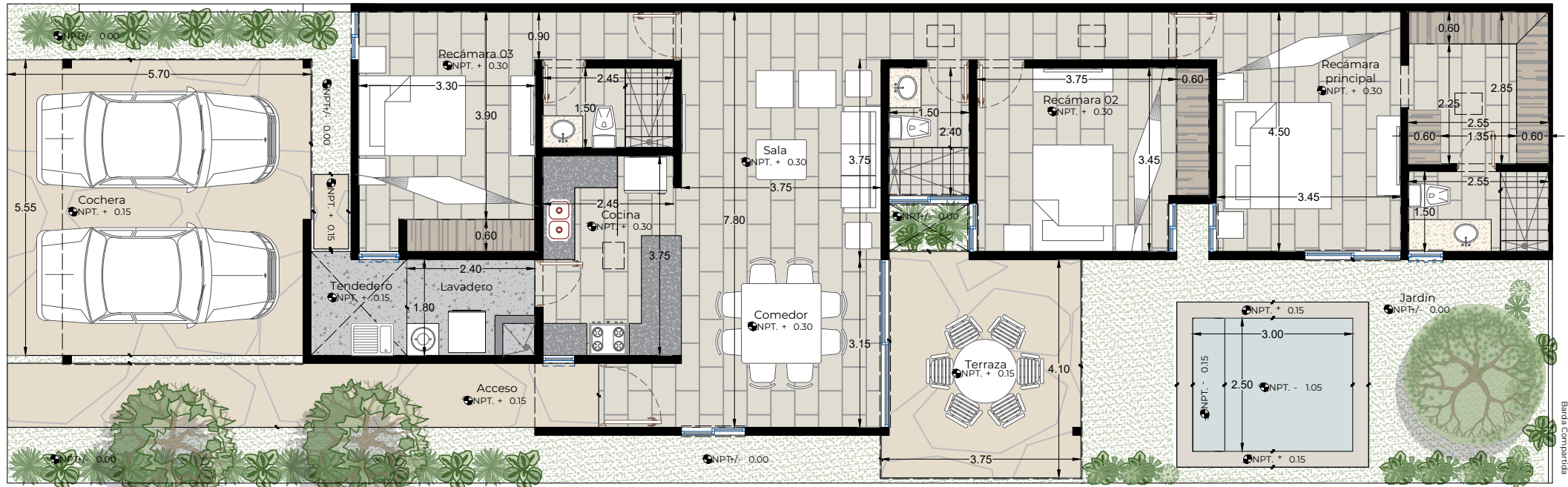
PLANTA BAJA
