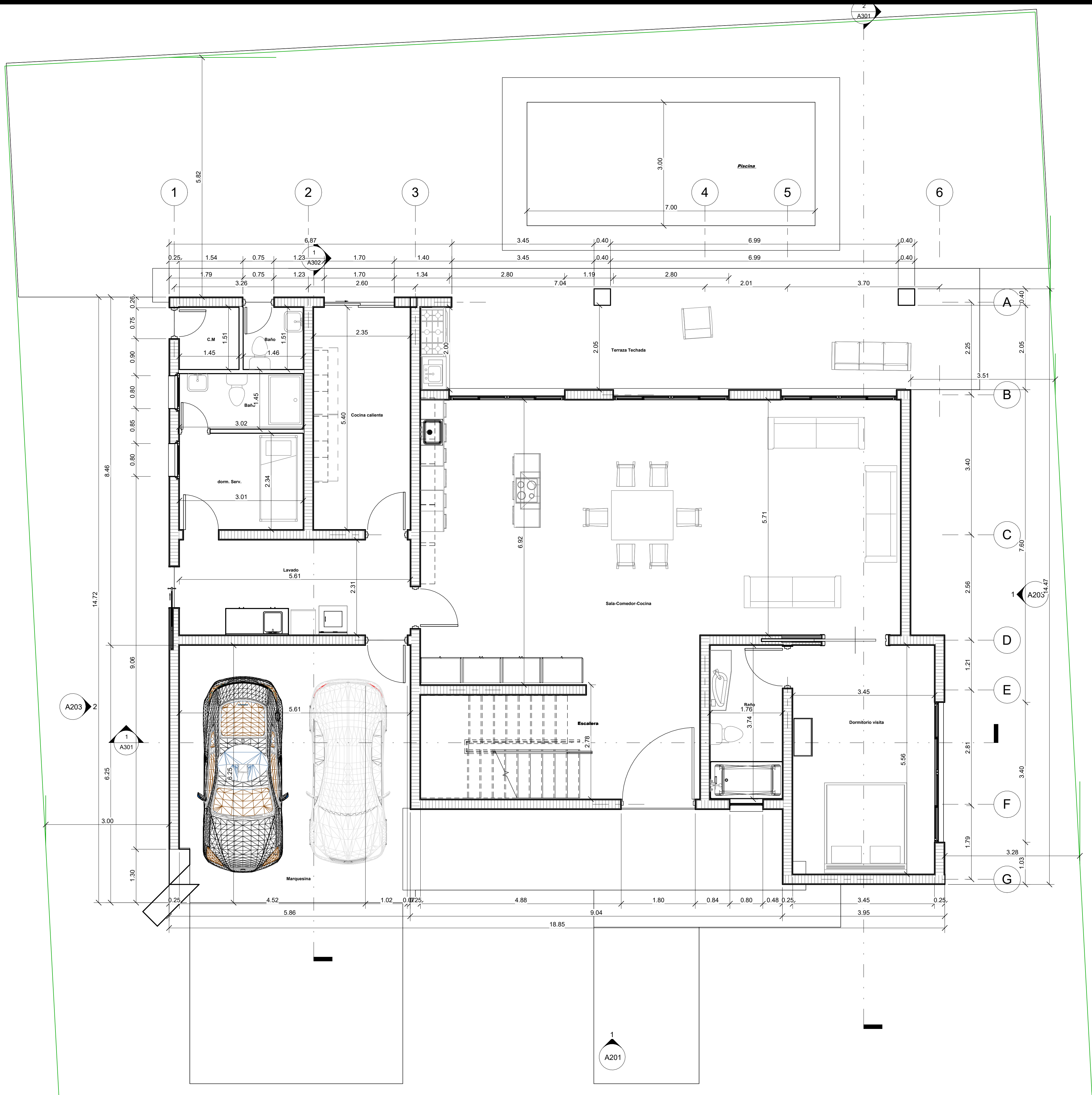
1 PLANTA DIMENSIONADA 1ER NIVEL 1 : 50
