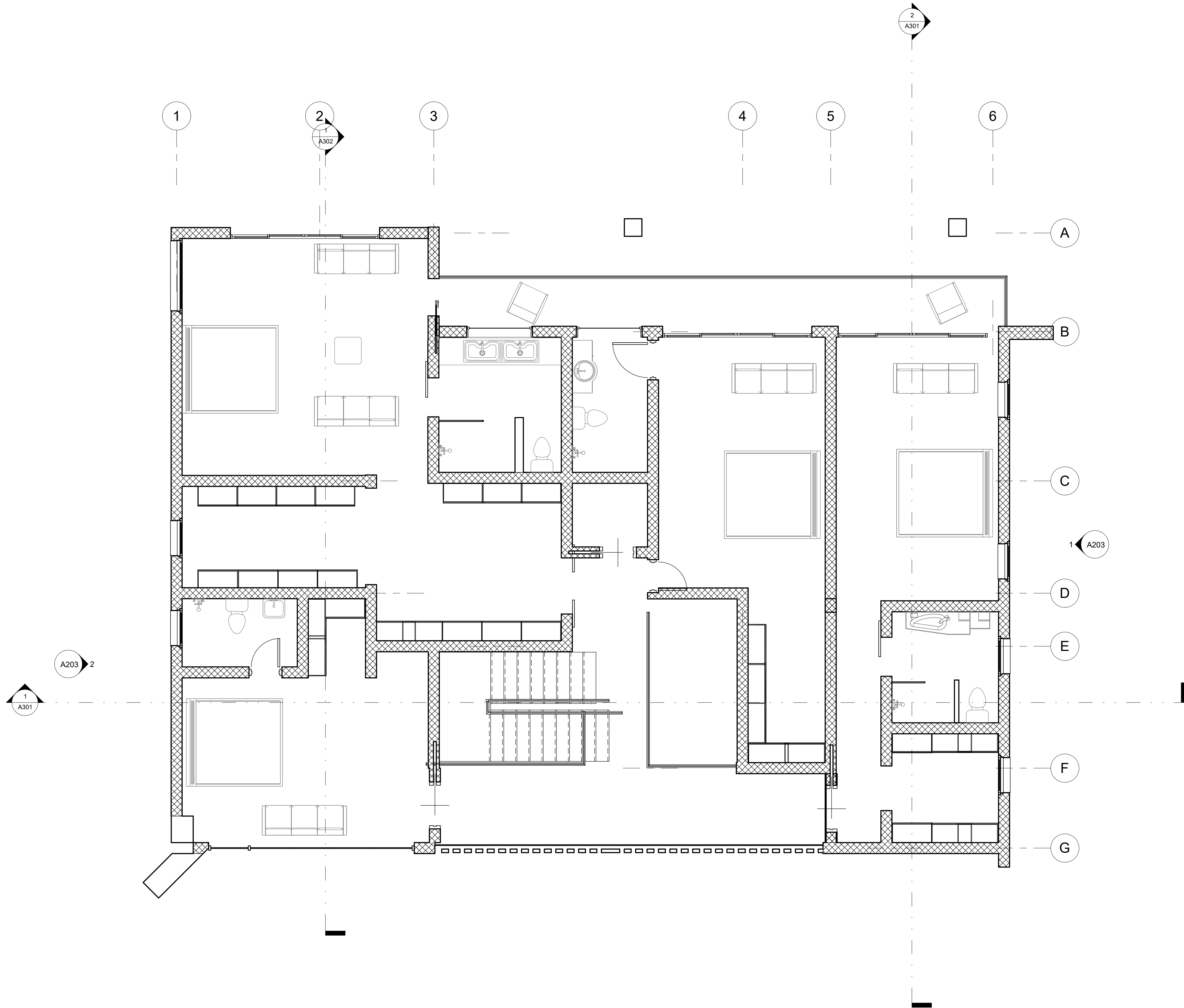
1 Planta Dim. 02 1 : 50
