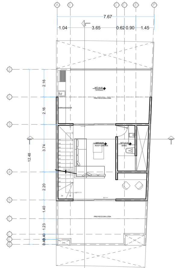
PLANTA SEGUNDO NIVEL
