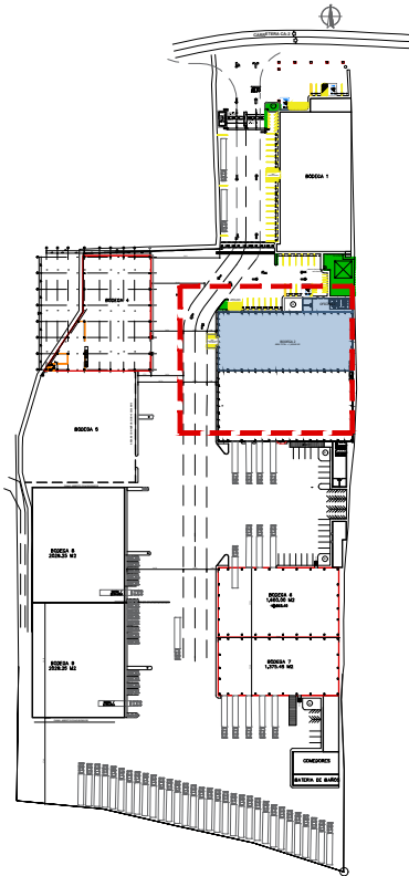
PLANTA GENERAL PROYECTO
