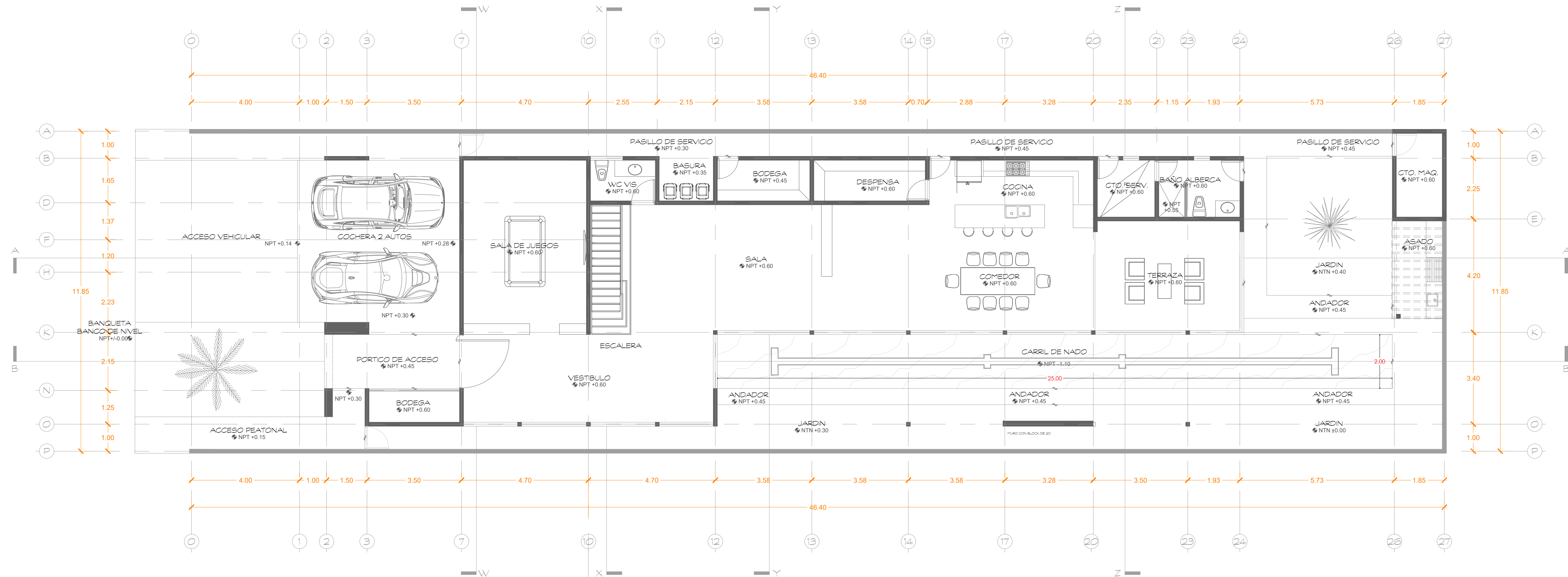
PLANTA BAJA
