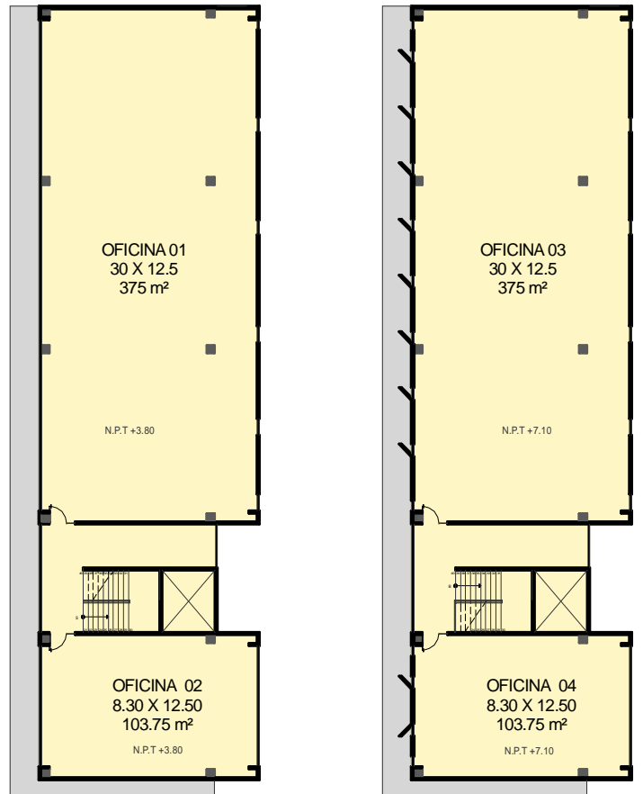
PLANTA ARQUITECTÓNICA SEGUNDO NIVEL N.P.T. +3.80
