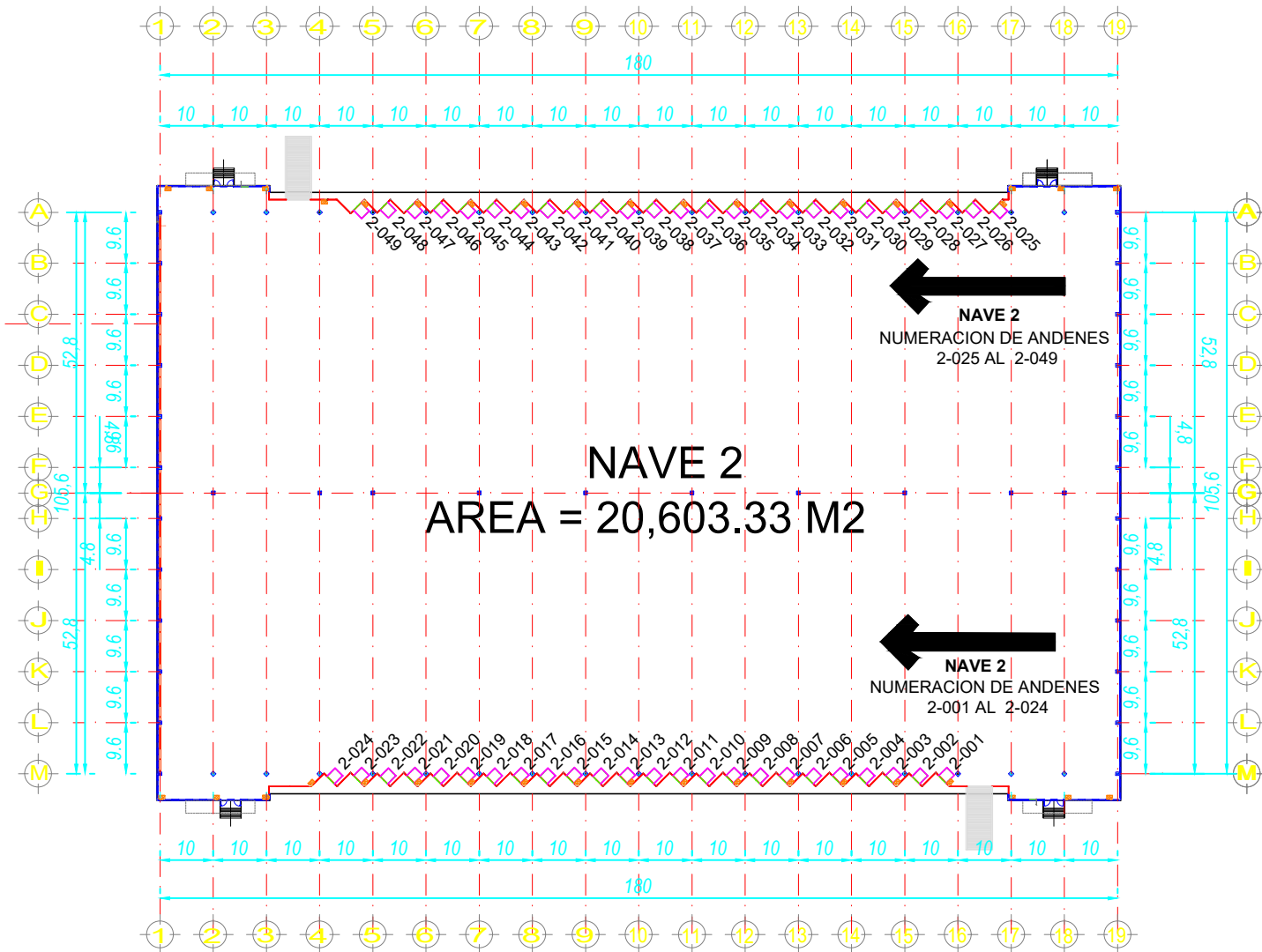
PLANTA ARQUITECTONICA NAVE 2
