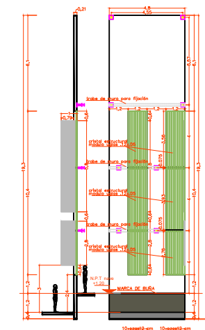
DETALLE MURO TIPO 4.80M
