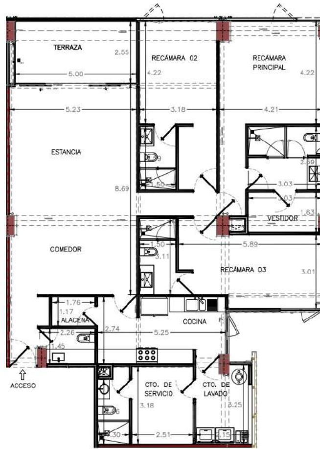
TIPO 03 ESC: 1:150
