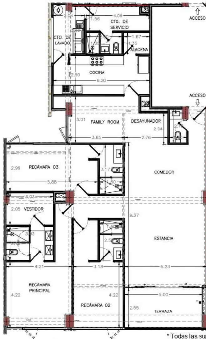
TIPO 01 ESC: 1:150
