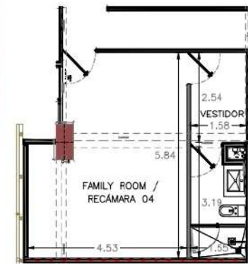
Opción recámara 04 ESC: 1:150
