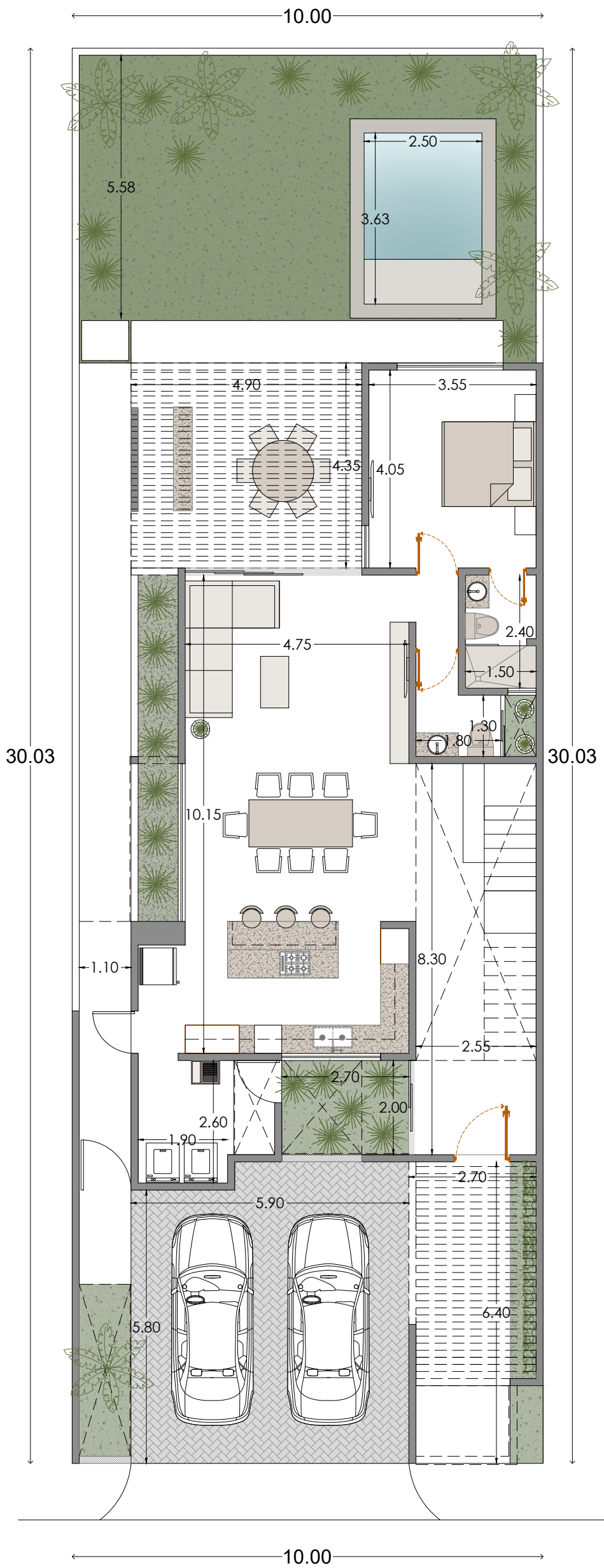
PLANTA BAJA
