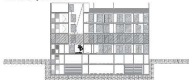
PLANTA N1
